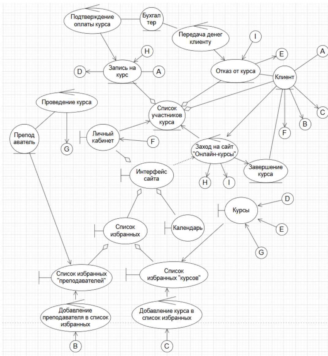
Рисунок 1 – Итоговая UML-модель системы согласно персональному варианту
