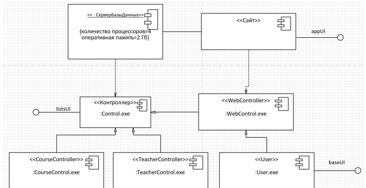
Рисунок 1 – Диаграмма компонентов персонального варианта
