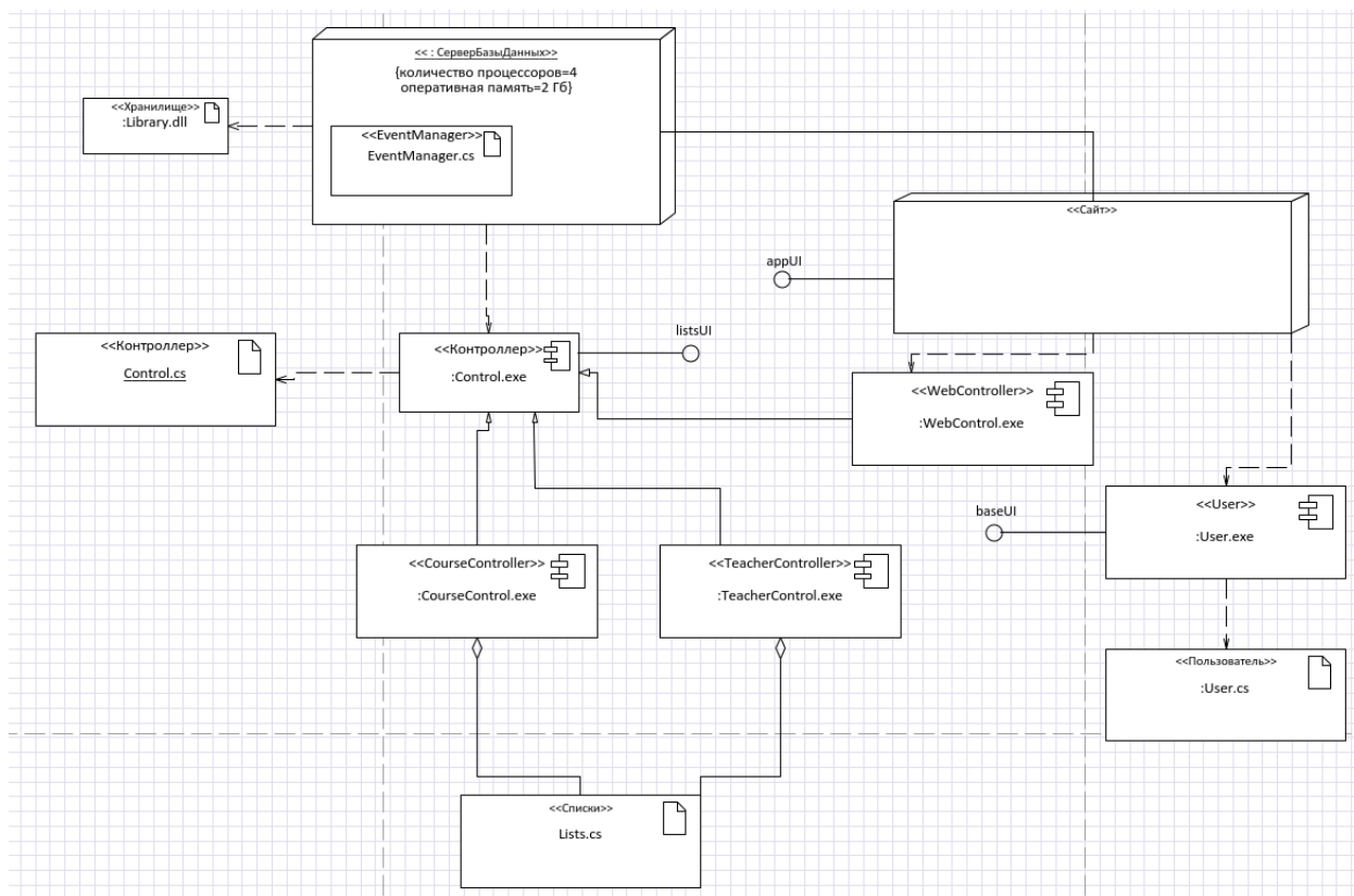
Рисунок 2 – Диаграмма развёртывания персонального варианта
