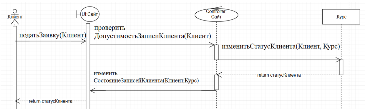
Рисунок 3 - Диаграмма последовательности по персональному варианту
