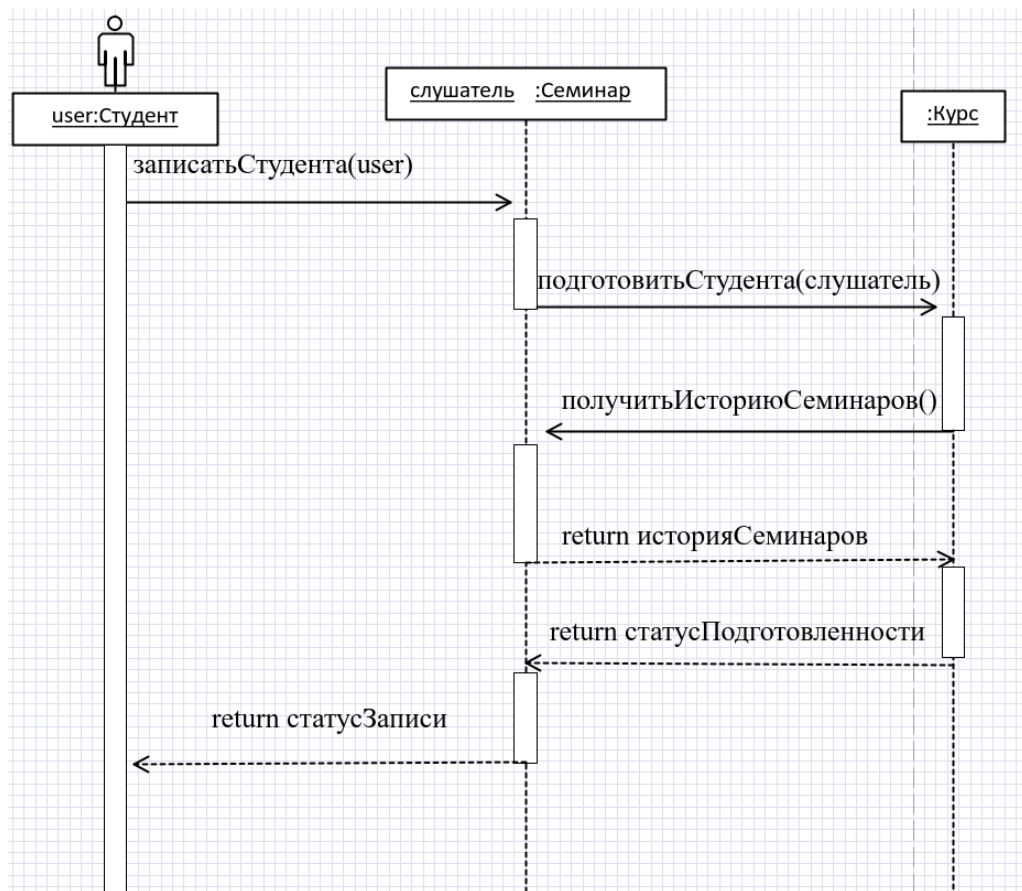
Рисунок 1 – Диаграмма последовательности для первого задания
