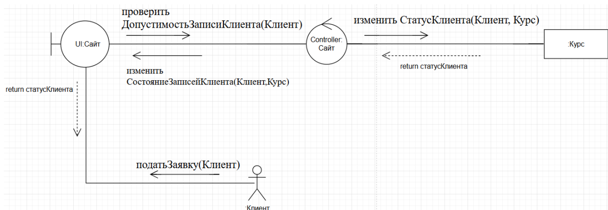
Рисунок 4 - Диаграмма кооперации по персональному варианту
