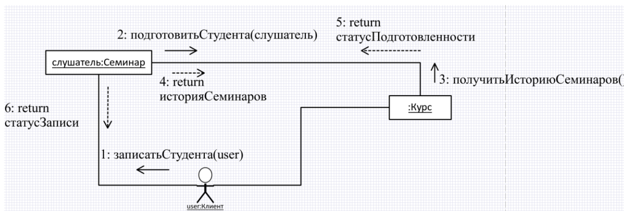
Рисунок 2 – Диаграмма кооперации для первого задания
