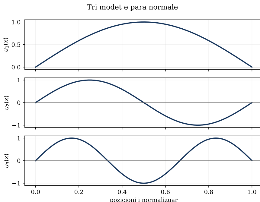
Figura 3.2: Mode normale të një sistemi njëpërmasor me skaje të fiksuara.
