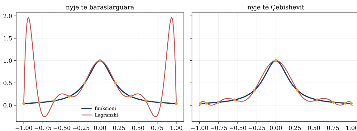
Figura 4.1: Interpolimi i funksionit Runge. Nyjet e Çebishevit zvogëlojnë lëkundjet në skaje.
