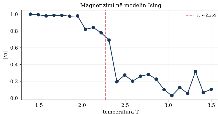
Figura 12.2: Rënia e magnetizimit pranë zonës kritike në një simulim të fundmë.
