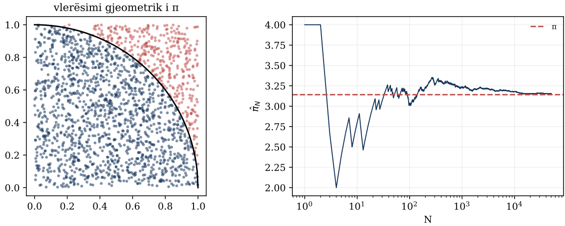
Figura 10.1: Vlerësimi gjeometrik i \pi dhe konvergjenca e vlerësuesit.
