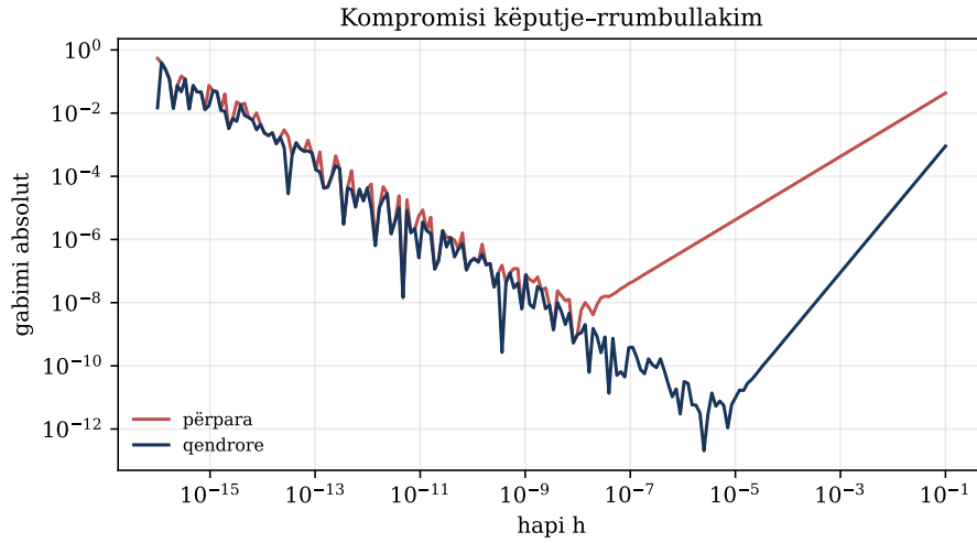
Figura 5.1: Gabimi total ka formë U: këputja dominon për hapa të mëdhenj, rrumbullakimi për hapa tepër të vegjël.
