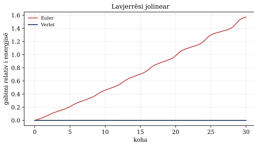
Figura 6.1: Euler-i krijon drift energjie, ndërsa Verlet ruan më mirë strukturën afatgjatë.
