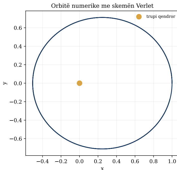
Figura 6.2: Orbitë e integruar me skemë simplektike.
