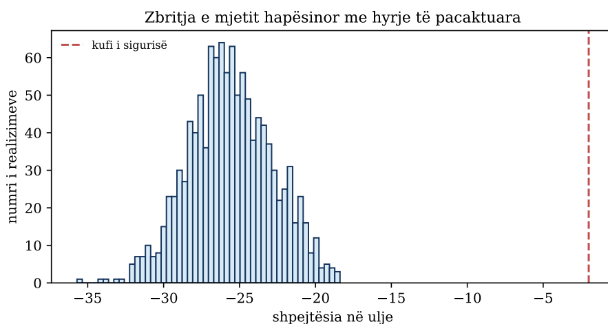
Figura 10.3: Shpërndarja e shpejtësisë së uljes kur lartësia, shpejtësia fillestare dhe shtytja kanë pacaktueshmëri.
