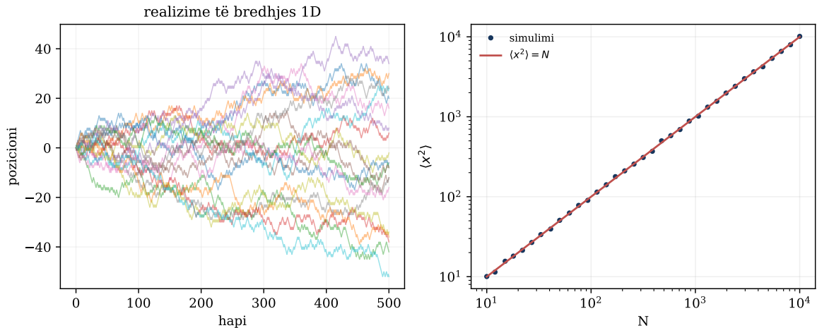
Figura 11.1: Realizime të bredhjes dhe rritja lineare e zhvendosjes katrore mesatare.
