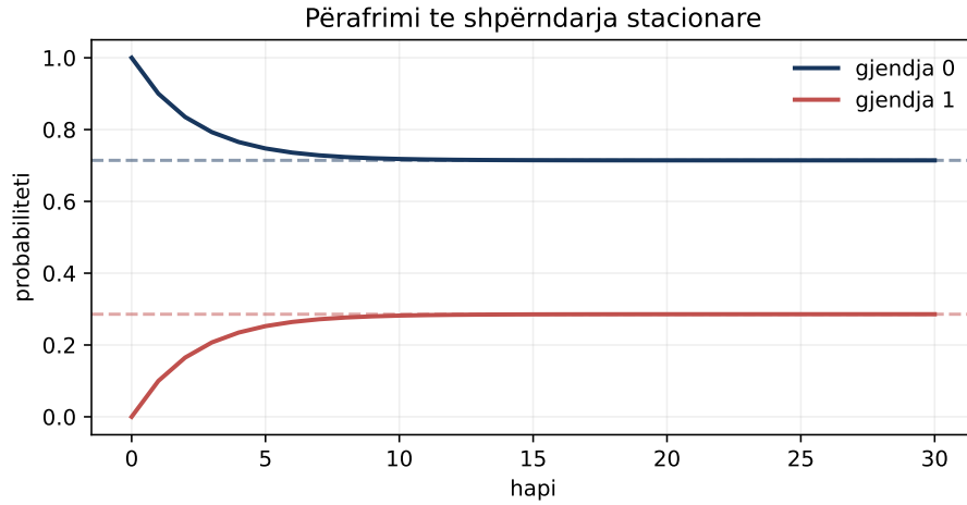
Figura 11.3: Humbja graduale e kujtesës së gjendjes fillestare në një zinxhir me dy gjendje.
