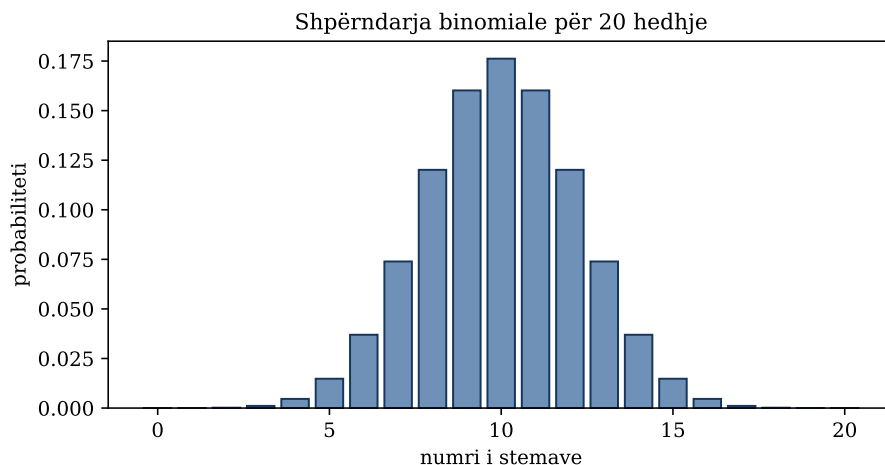
Figura 8.1: Shpërndarja e numrit të stemave në 20 hedhje të një monedhe të paanshme.
