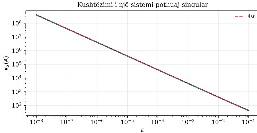
Figura 2.2: Rritja e numrit të kushtëzimit kur dy rreshta të matricës bëhen pothuaj linearë të varur.
