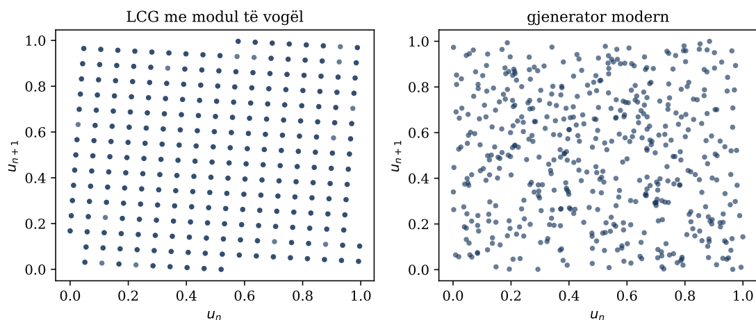
Figura 9.1: Grafiku (u_n, u_{n+1}) zbulon strukturë rrjete në një gjenerator të dobët.
