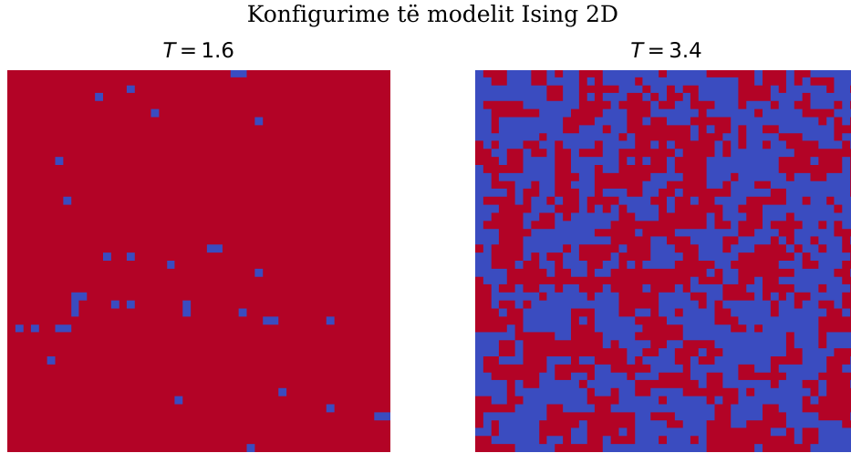
Figura 12.1: Formimi i domeneve nën temperaturën kritike dhe çrregullimi sipër saj.
