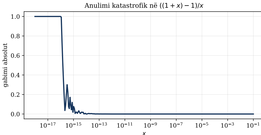
Figura 2.1: Gabimi i shkaktuar nga anulimi kur x bëhet i krahasueshëm me saktësinë e makinës.
