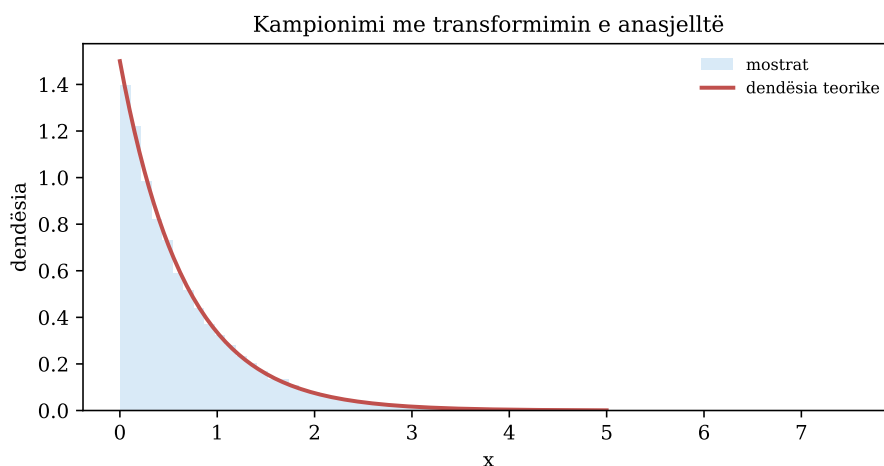
Figura 9.2: Mostrat e gjeneruara me transformimin e anasjelltë dhe dendësia teorike.
