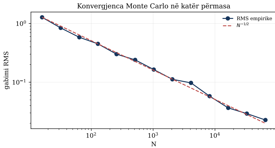
Figura 10.2: Shkallëzimi N^{-1/2} në një integral katërpërmasor.
