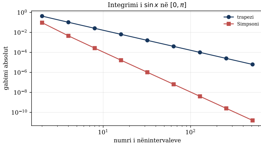
Figura 5.2: Konvergjencia e trapezit dhe Simpsonit për një integral me zgjidhje të njohur.
