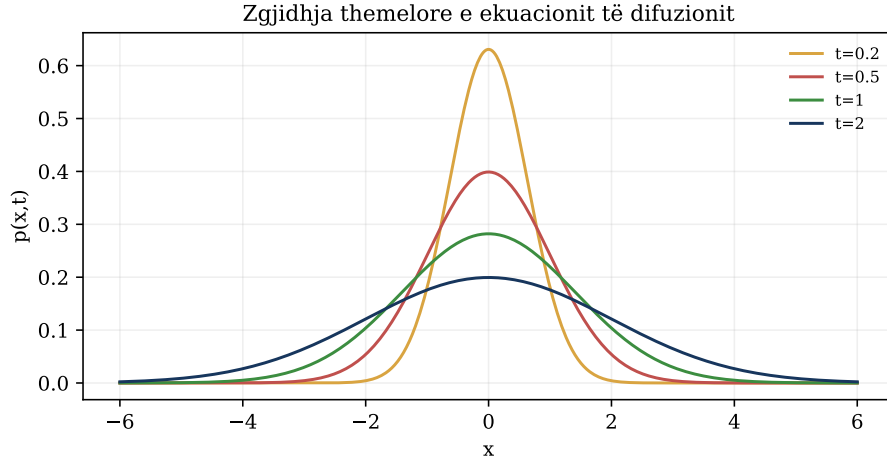
Figura 11.2: Profili i difuzionit zgjerohet, ndërsa normalizimi ruhet.
