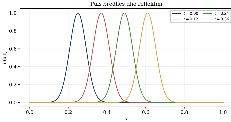
Figura 7.1: Evolucioni i një pulsi bredhës dhe përafrimi te kufiri reflektues.
