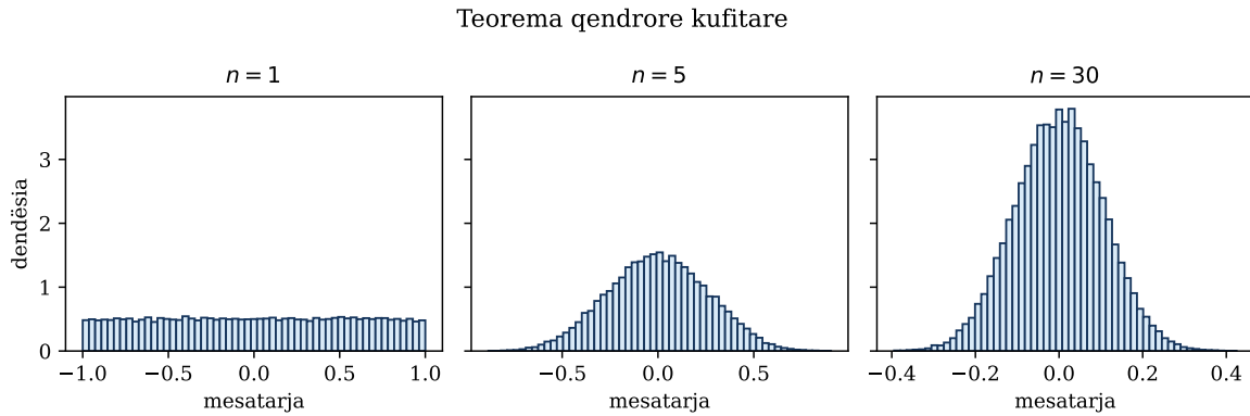
Figura 8.2: Shpërndarja e mesatares së ndryshoreve uniforme afrohet me formën Gauss kur rritet numri i termave.
