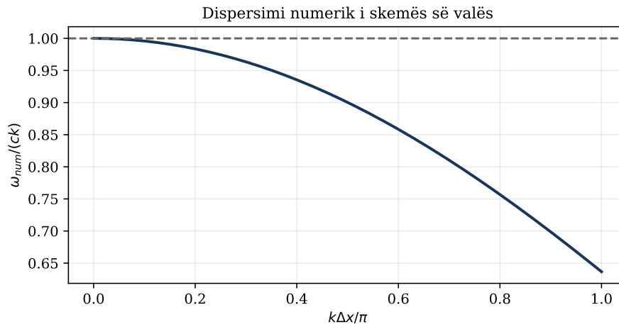
Figura 7.2: Shpejtësia fazore numerike zvogëlohet për numra valorë të lartë.
