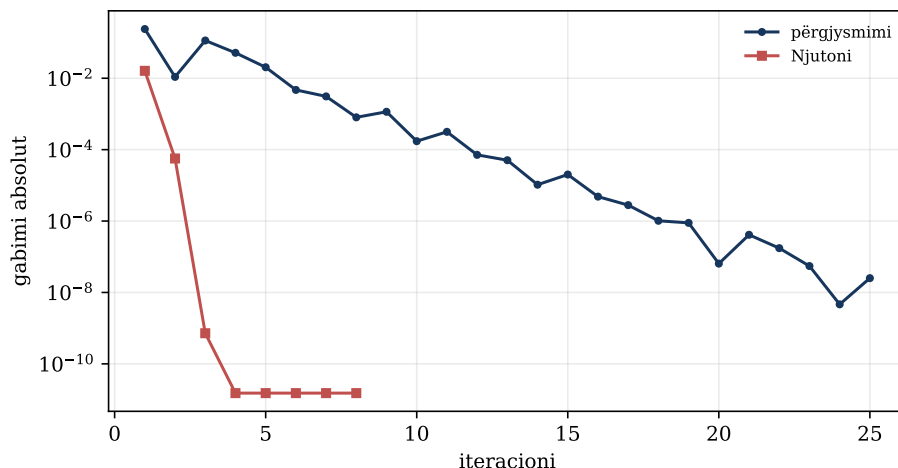
Figura 3.1: Konvergjenca lineare e përgjysmimit dhe konvergjenca e shpejtë e Njutonit për \cos x - x = 0 .
