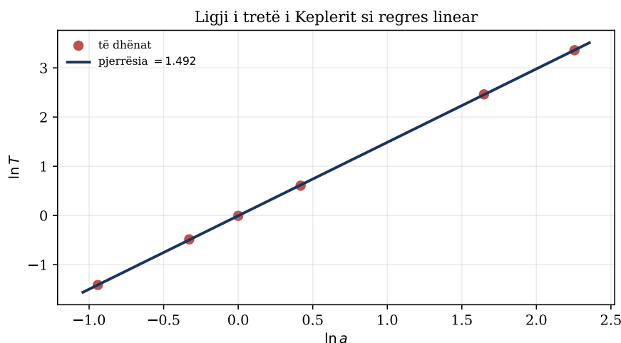
Figura 4.2: Linearizimi logarithmik i T^2 \propto a^3 . Pjerrësia e pritur për \ln T kundrejt \ln a është 3/2 .
