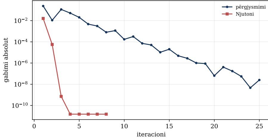
Figura 3.1: Konvergjencia lineare e përgjysmimit dhe konvergjencia e shpejtë e Njutonit për \cos x - x = 0 .
