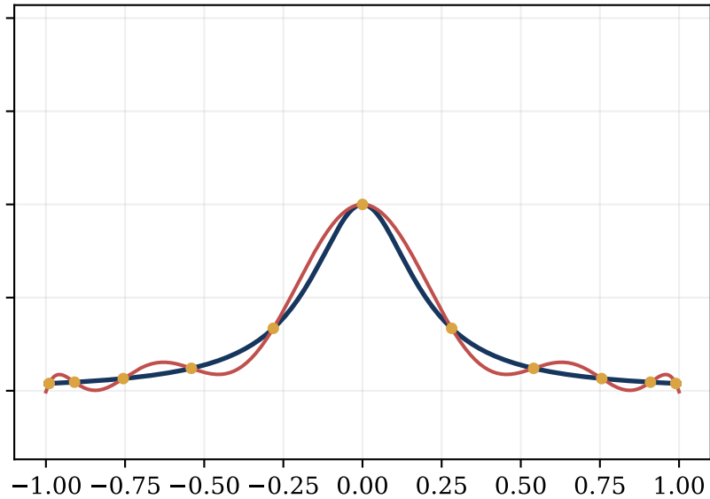
nyje të Çebishevit
