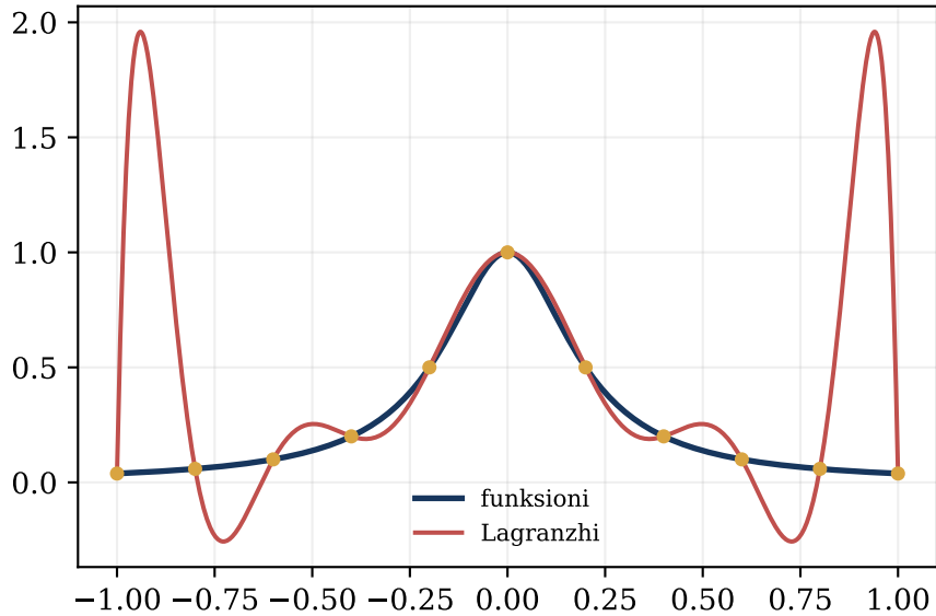
nyje të baraslarguara
