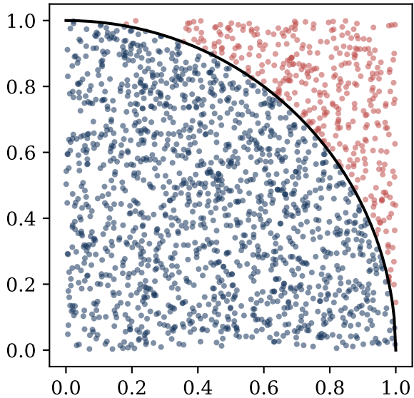
vlerësimi gjeometrik i \pi
