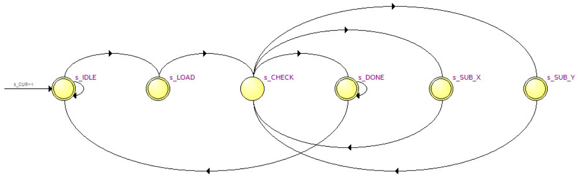
Figura 1 – Diagrama da máquina de estados exportado do Quartus Prime.
