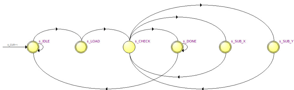
Figura 4 – FSM sintetizada pelo Quartus Prime, confirmando a implementação VHDL.
