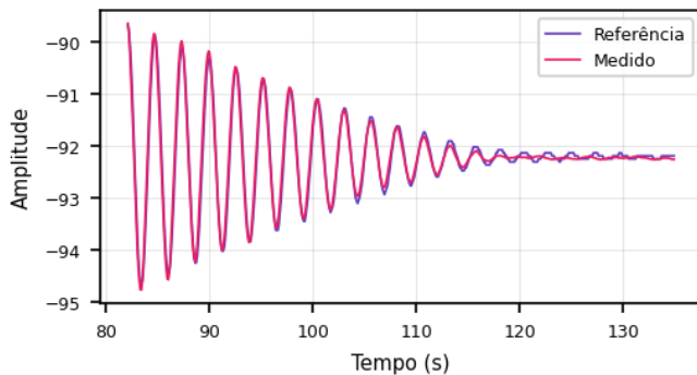
Roll: Referência vs. Medido (99.94%)
