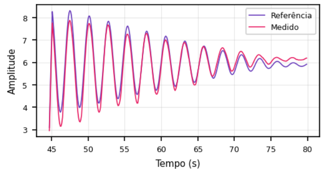
Pitch: Referência vs. Medido (99.28%)
