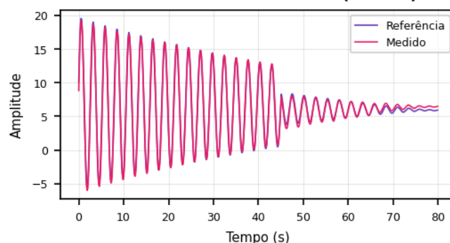
Pitch: Referência vs. Medido (99.16%)
