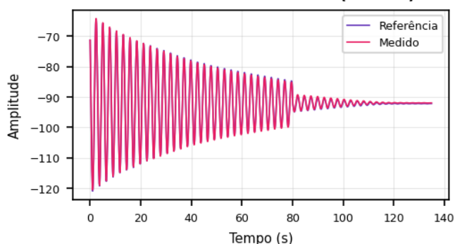
Roll: Referência vs. Medido (99.87%)
