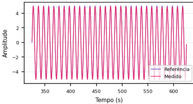
Roll: Referência vs. Medido (99.31%)
