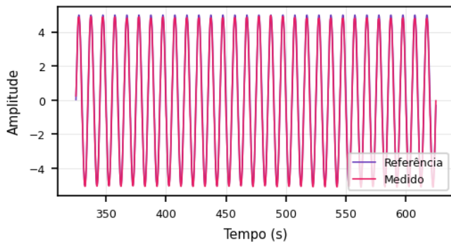
Roll: Referência vs. Medido (99.13%)
