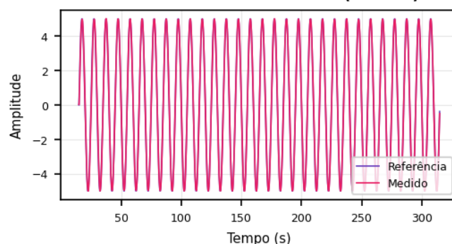
Pitch: Referência vs. Medido (99.93%)
