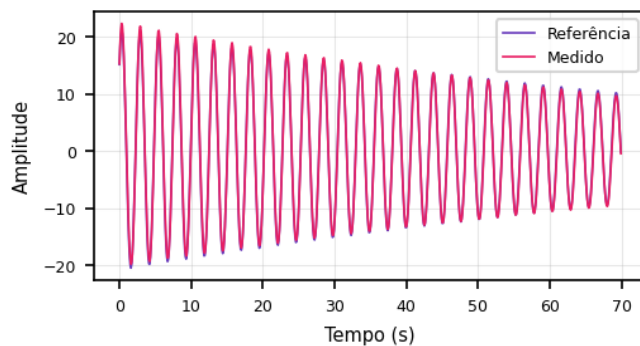
Pitch: Referência vs. Medido (99.76%)
