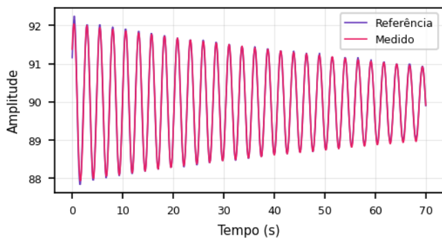
Roll: Referência vs. Medido (99.78%)
