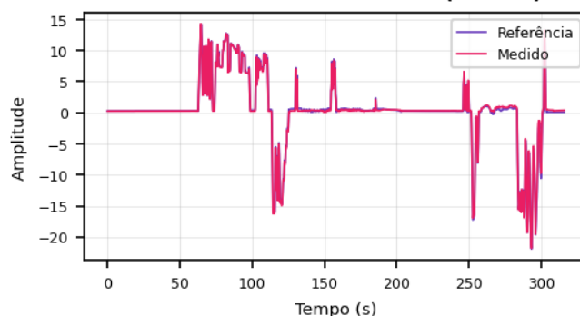
Pitch: Referência vs. Medido (99.29%)
