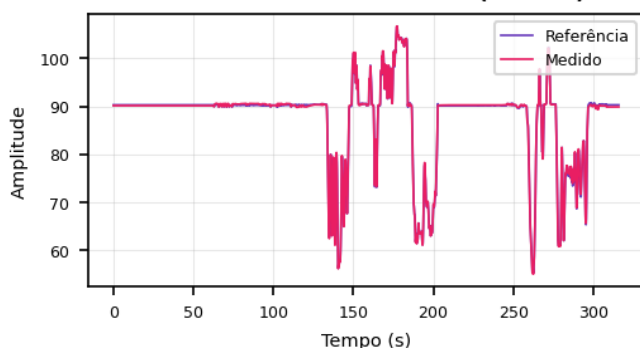
Roll: Referência vs. Medido (99.66%)
