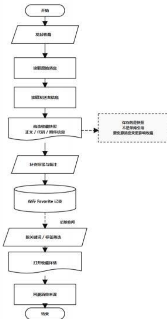
图 4.8 收藏流程图
