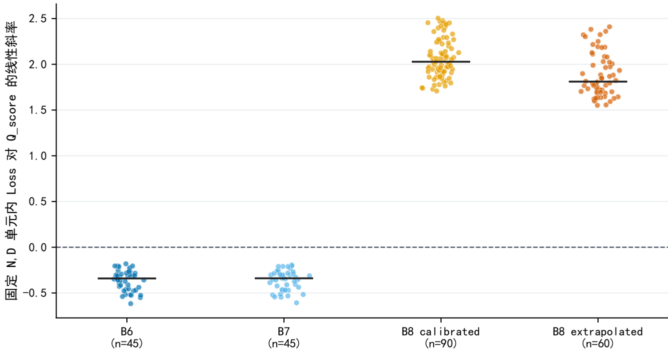
固定 N, D 后, B8 与 B6/B7 的 Q 方向相反
