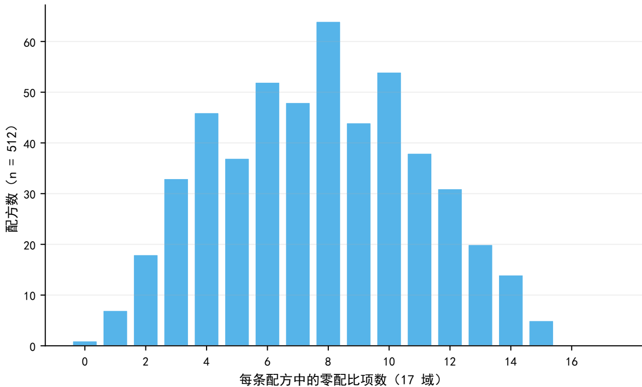
A4 零配比稀疏度；511/512 条配方至少含一个零
