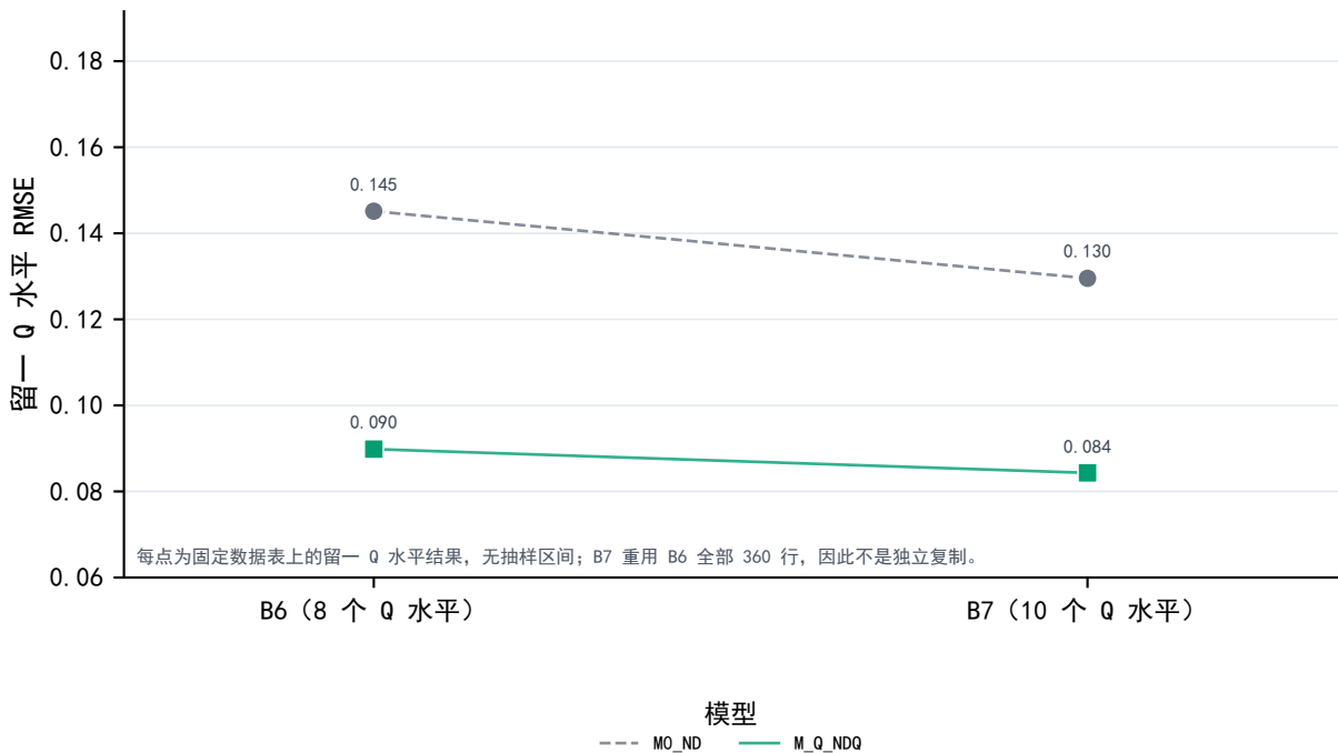
半合成网格中的条件模型比较
