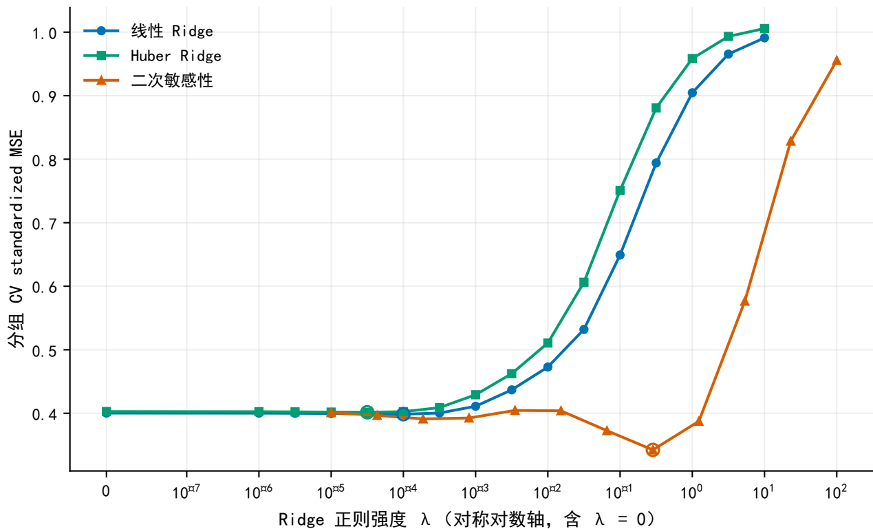
A4/A5 训练内正则强度选择；空心点为各模型最低分
