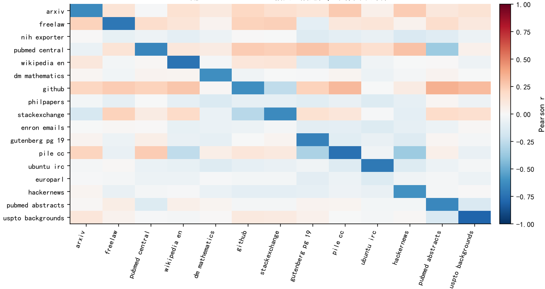
A4/A5 配比—Loss Pearson 相关（描述性，不作因果解释）
