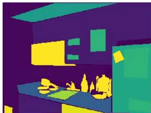
SemSeg (GT)
