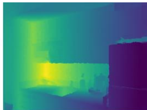
Depth (GT)
