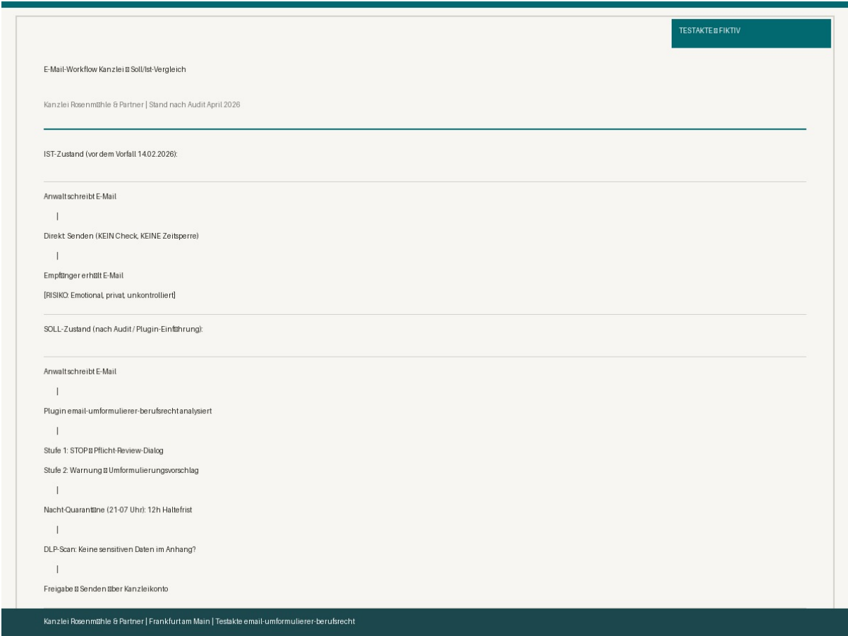
Bilddatei: email_workflow_kanzlei_diagramm.jpg
