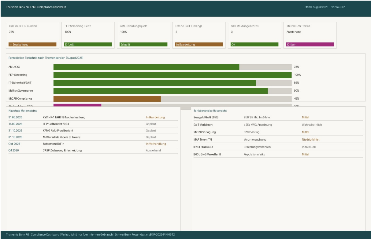
Bilddatei: compliance-dashboard-screenshot.jpg
