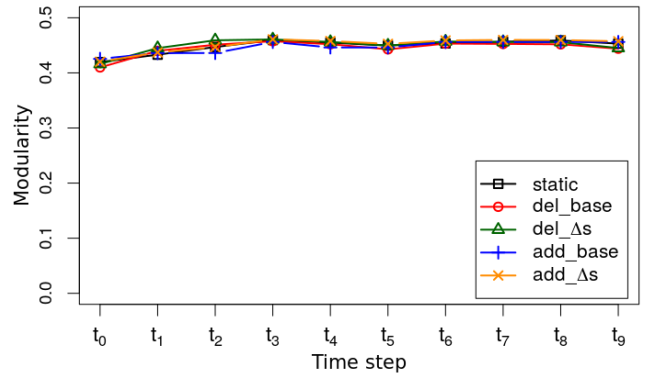
(d) Modularity for sx-stackoverflow+,sx-stackoverflow- network
