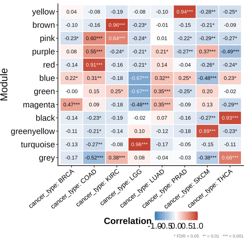
d Module-trait correlation
