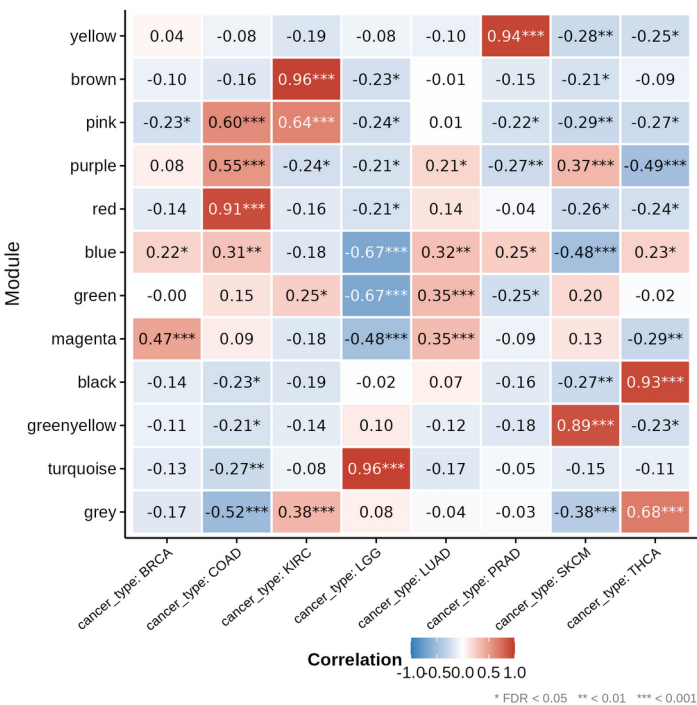
d Module-trait correlation
