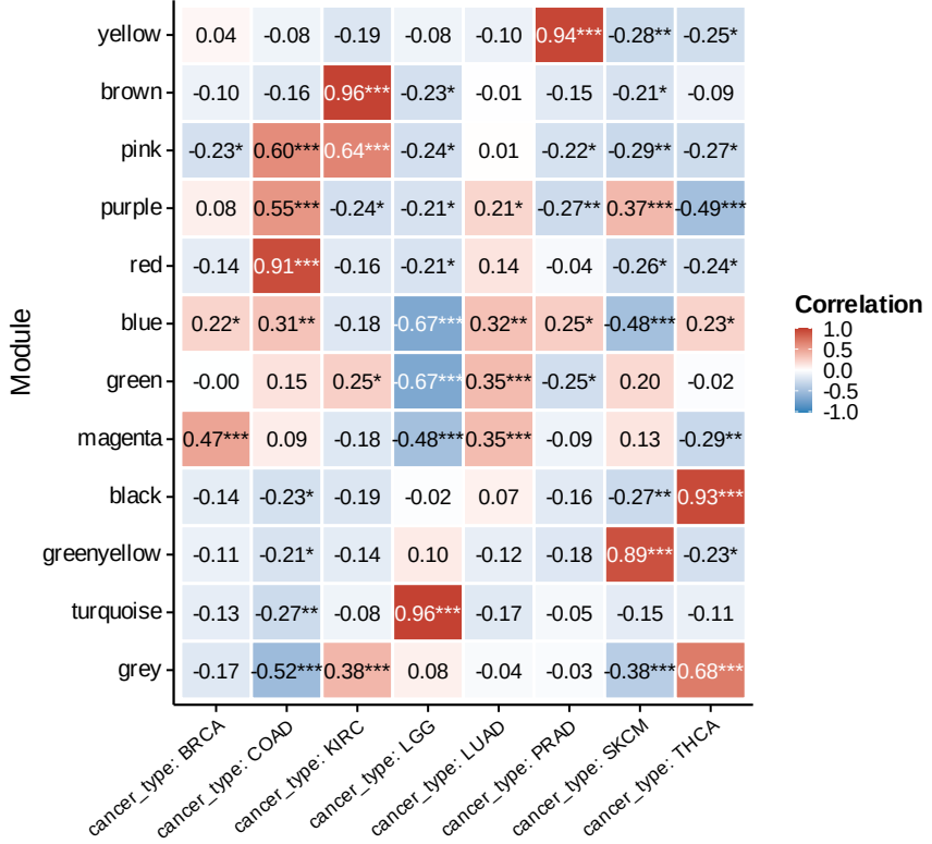
Module-trait correlation
