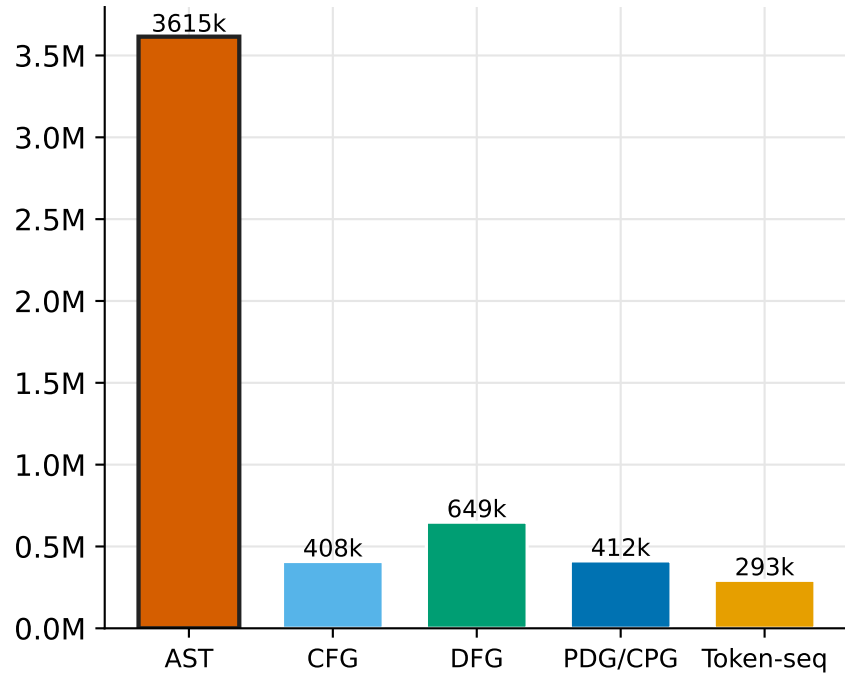
delta-edges per layer
