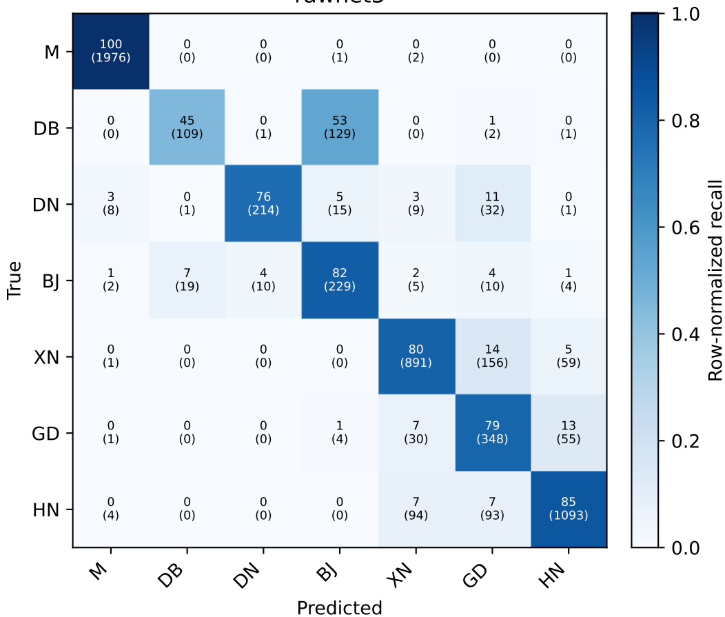
rawnet3
