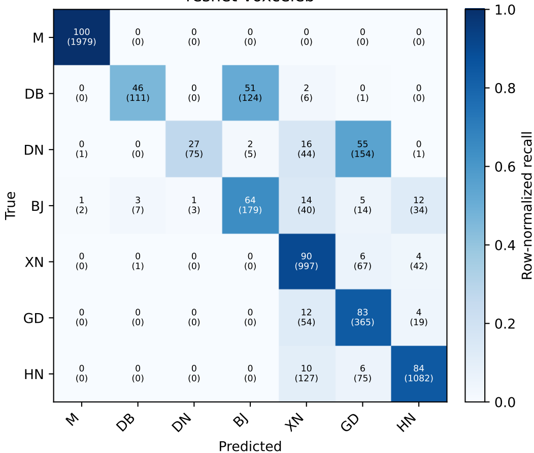
resnet-voxceleb
