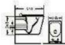
WH-028 مراجل على الحائط Wall-hung toilet Size: 510x345x340mm P-trap, 180mm roughing-in
