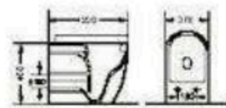
WH-003D مراجل على الحائط Floor mounted toilet Size: 550x370x400mm D-trap, 180mm
