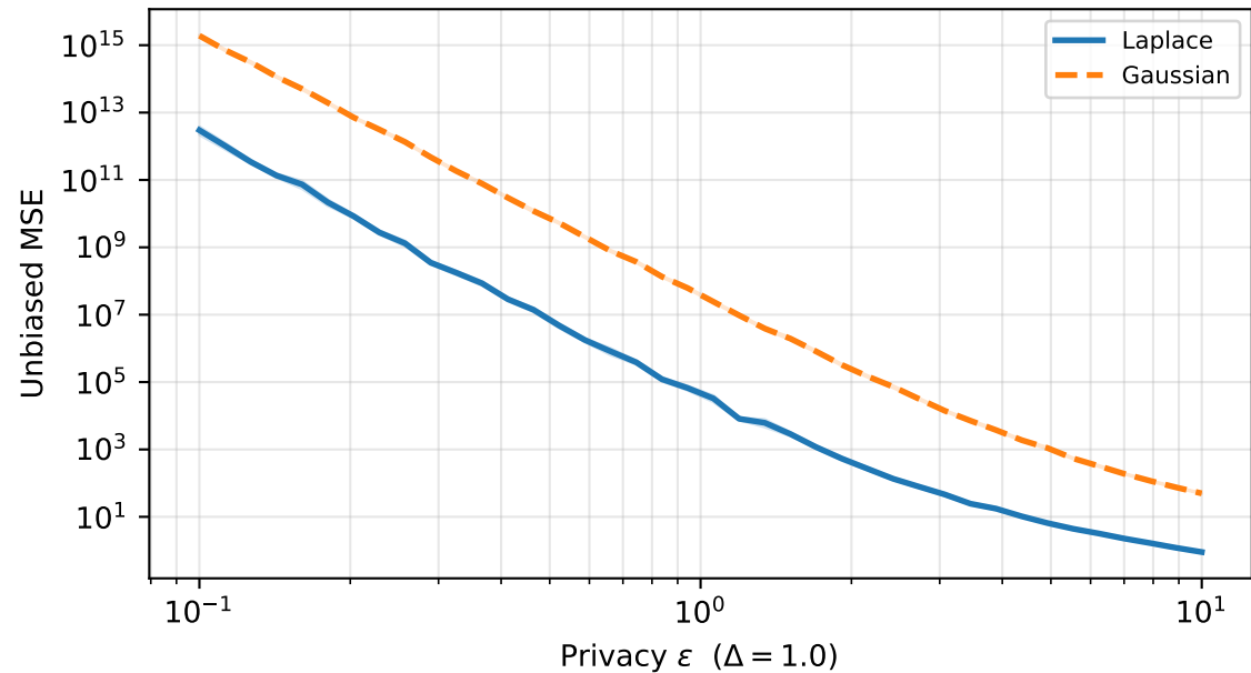
Unbiased MSE
