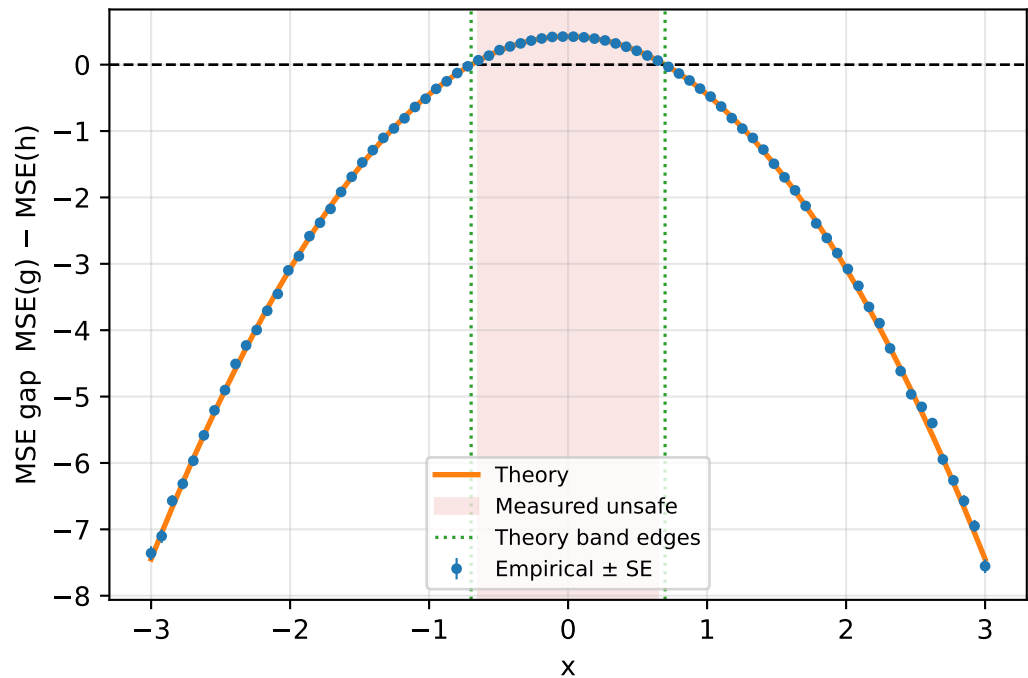
MSE gap
