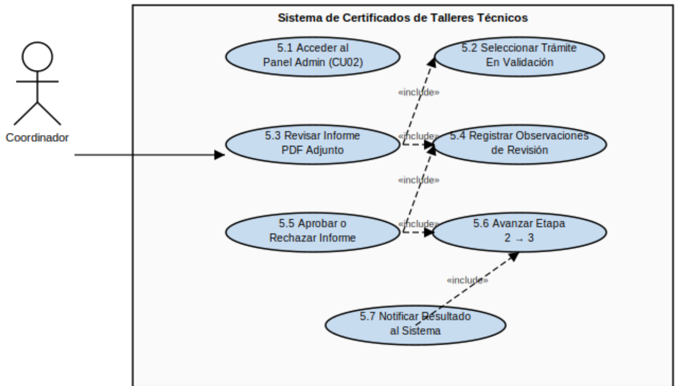
Figura 2.1: Diagrama de caso de uso de la HU 05
