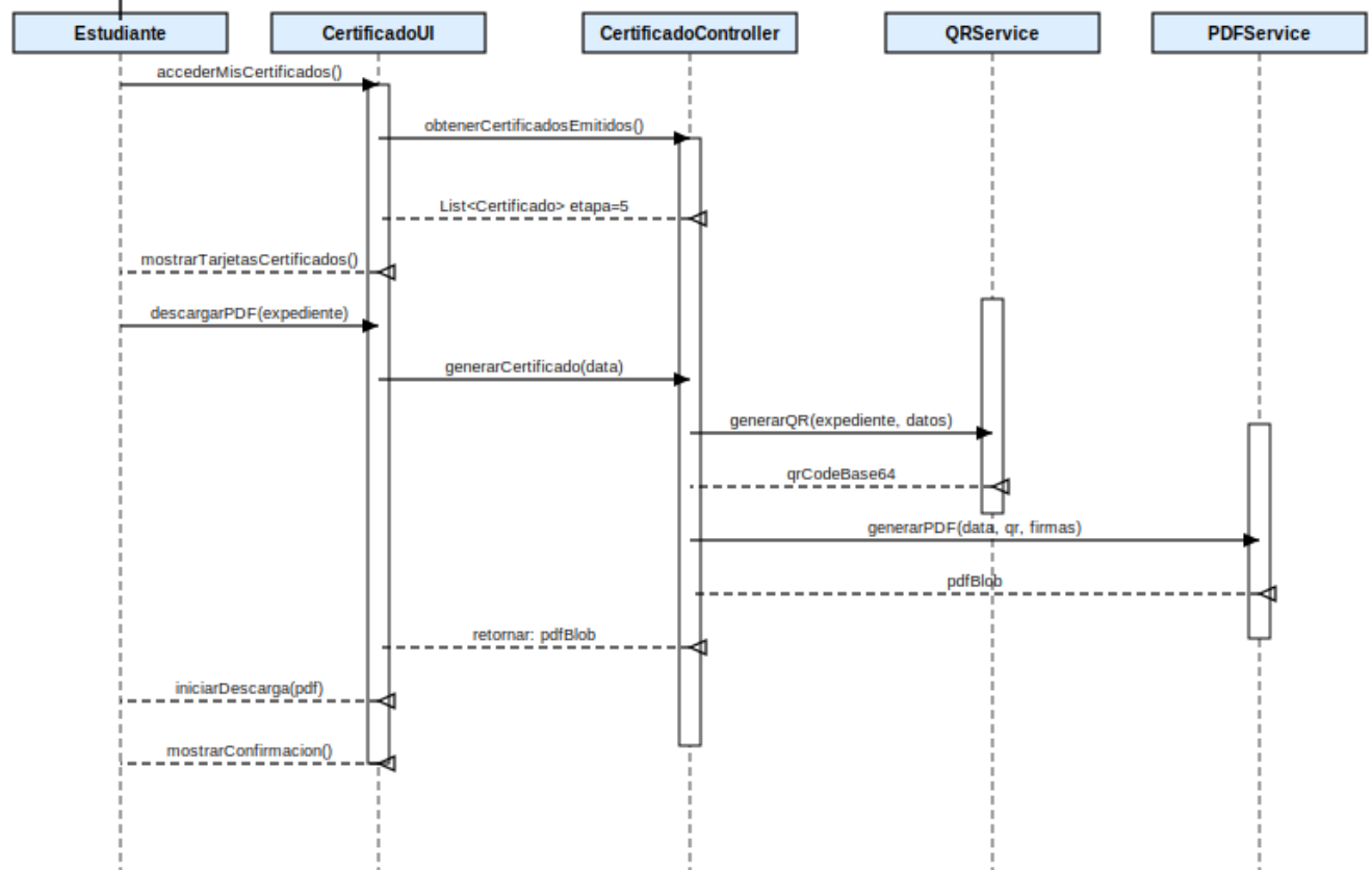
Figura 4.2: Diagrama de secuencia de la HU 09
