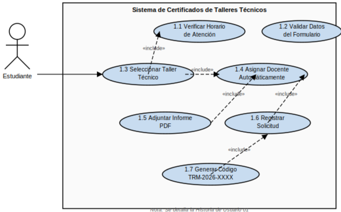
Figura 1.1: Diagrama de caso de uso de la HU 01
