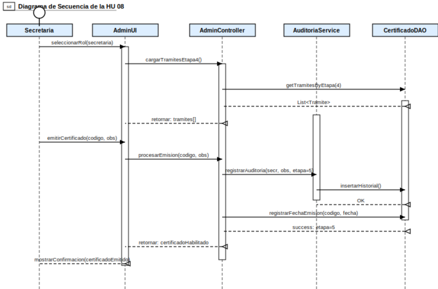
Figura 5.2: Diagrama de secuencia de la HU 08
