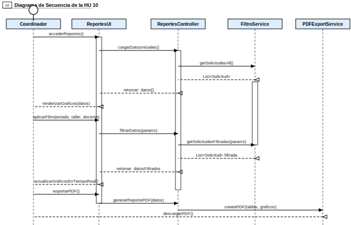
Figura 5.2: Diagrama de secuencia de la HU 10
