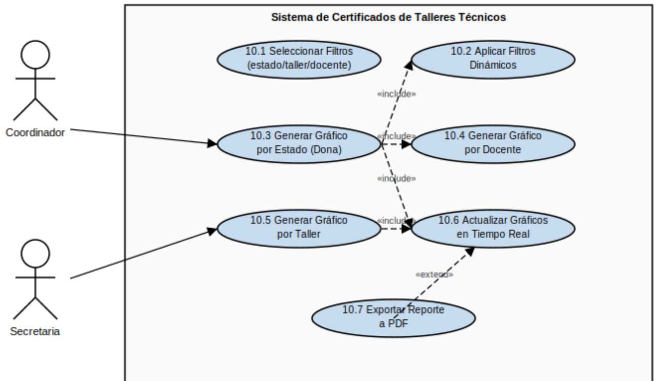
Figura 5.1: Diagrama de caso de uso de la HU 10
