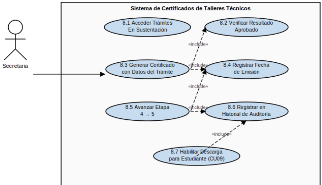
Figura 5.1: Diagrama de caso de uso de la HU 08
