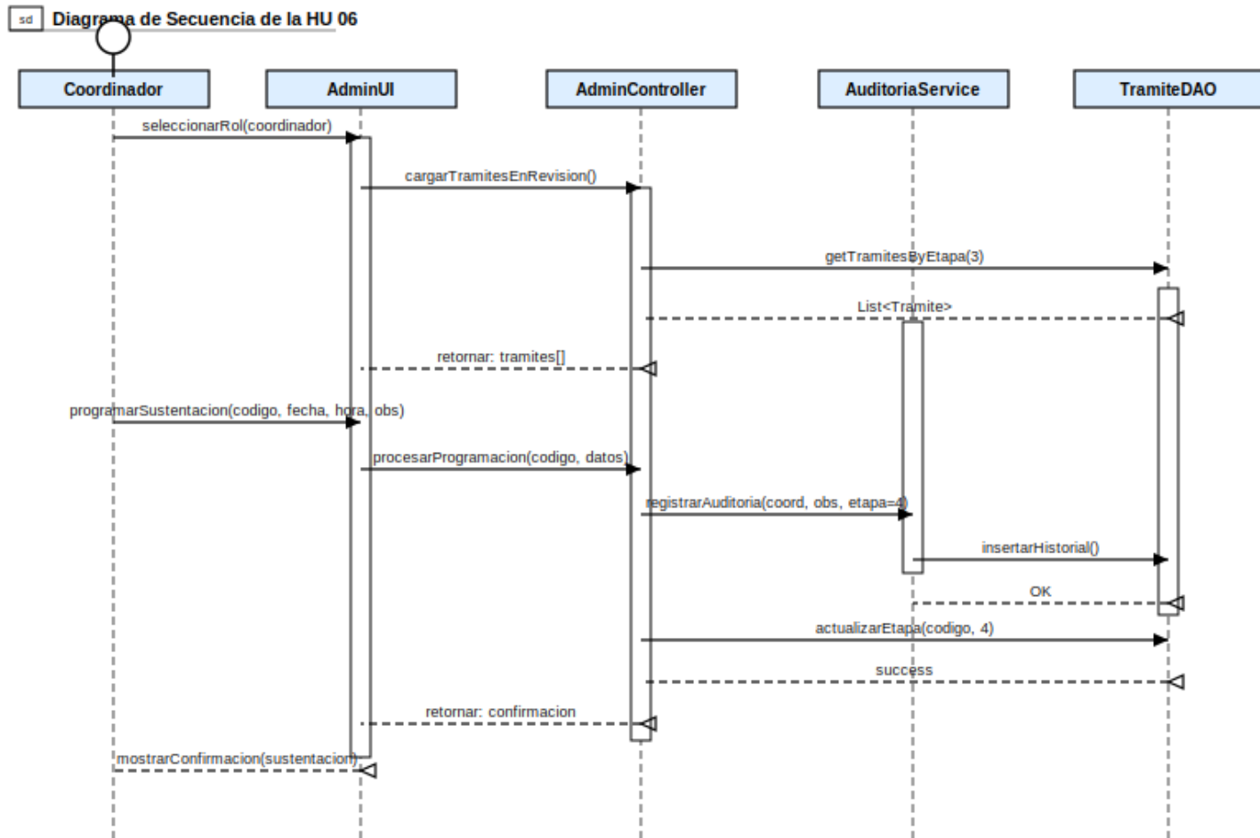
Figura 3.2: Diagrama de secuencia de la HU 06
