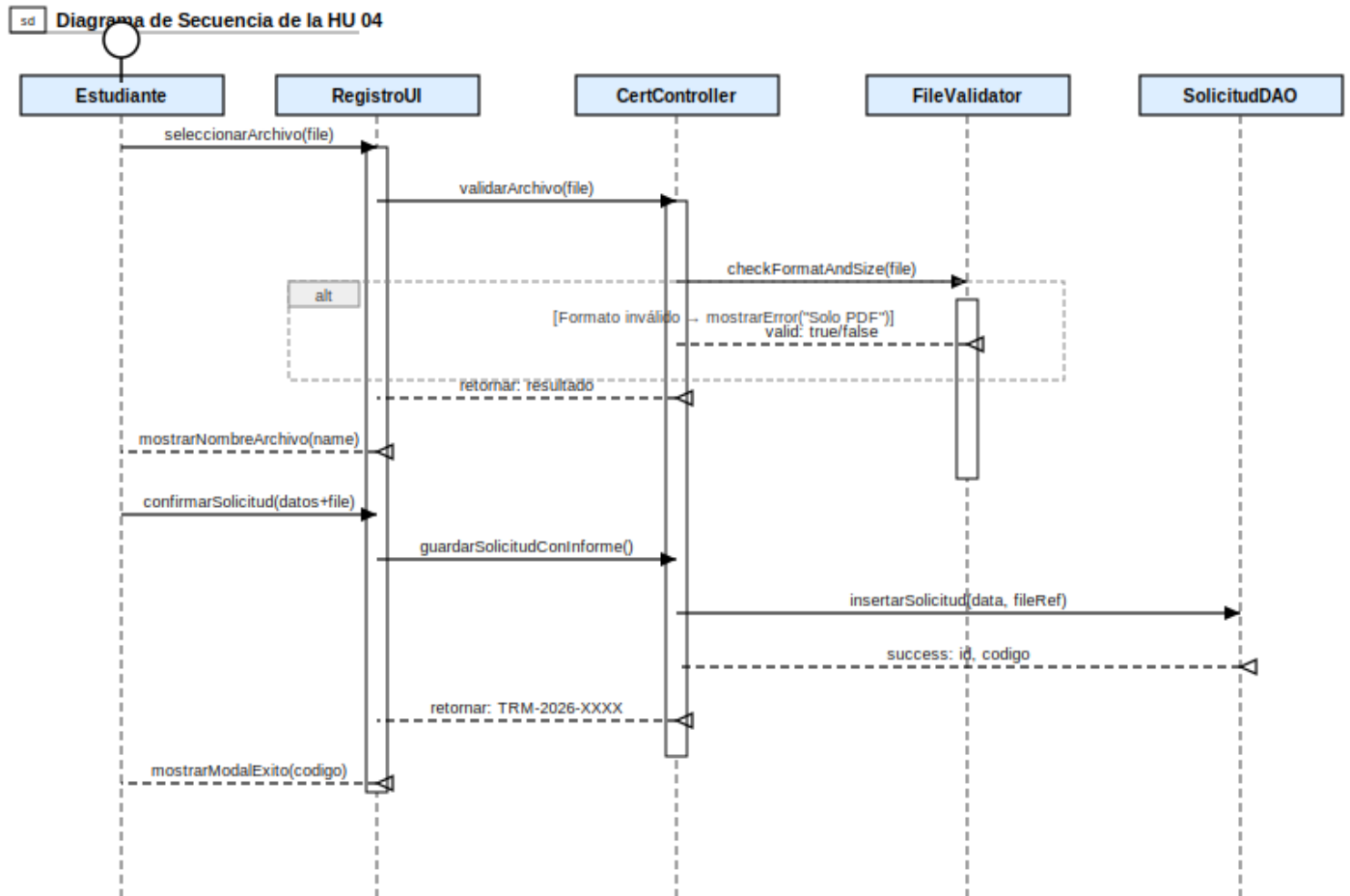
Figura 1.2: Diagrama de secuencia de la HU 04
