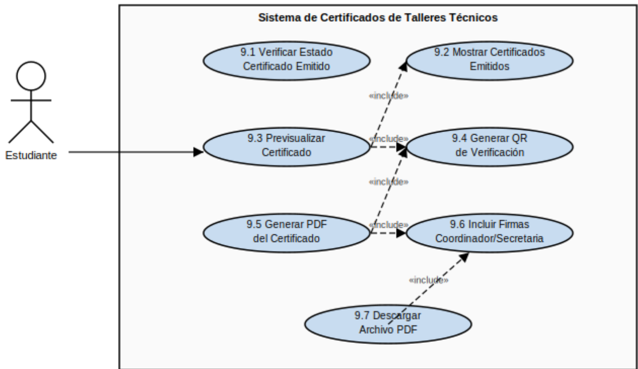
Figura 4.1: Diagrama de caso de uso de la HU 09
