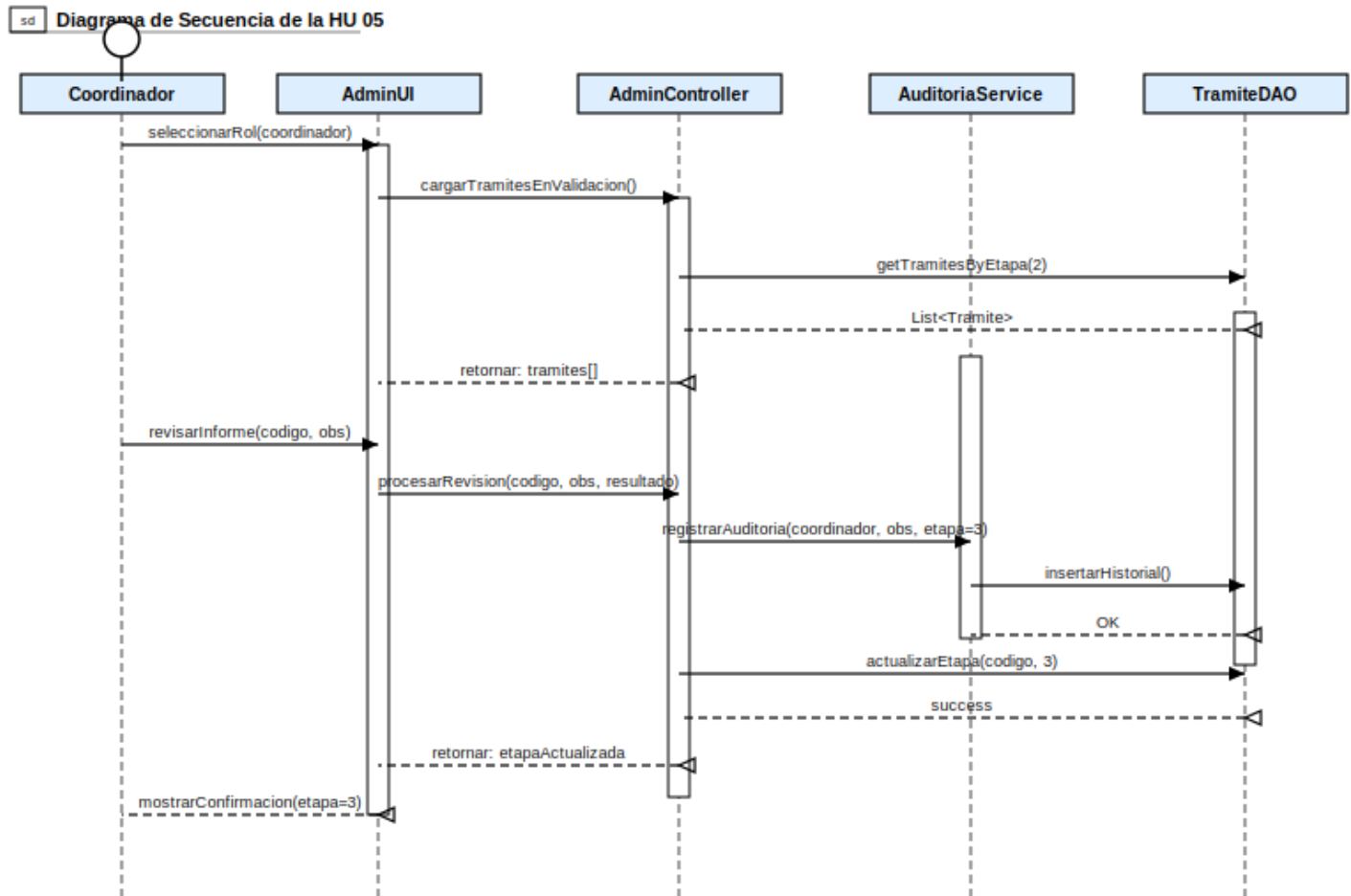
Figura 2.2: Diagrama de secuencia de la HU 05
