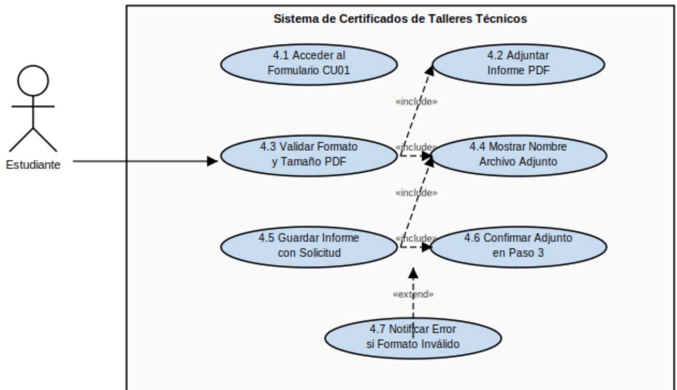
Figura 1.1: Diagrama de caso de uso de la HU 04
