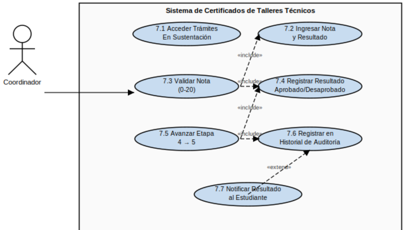
Figura 4.1: Diagrama de caso de uso de la HU 07
