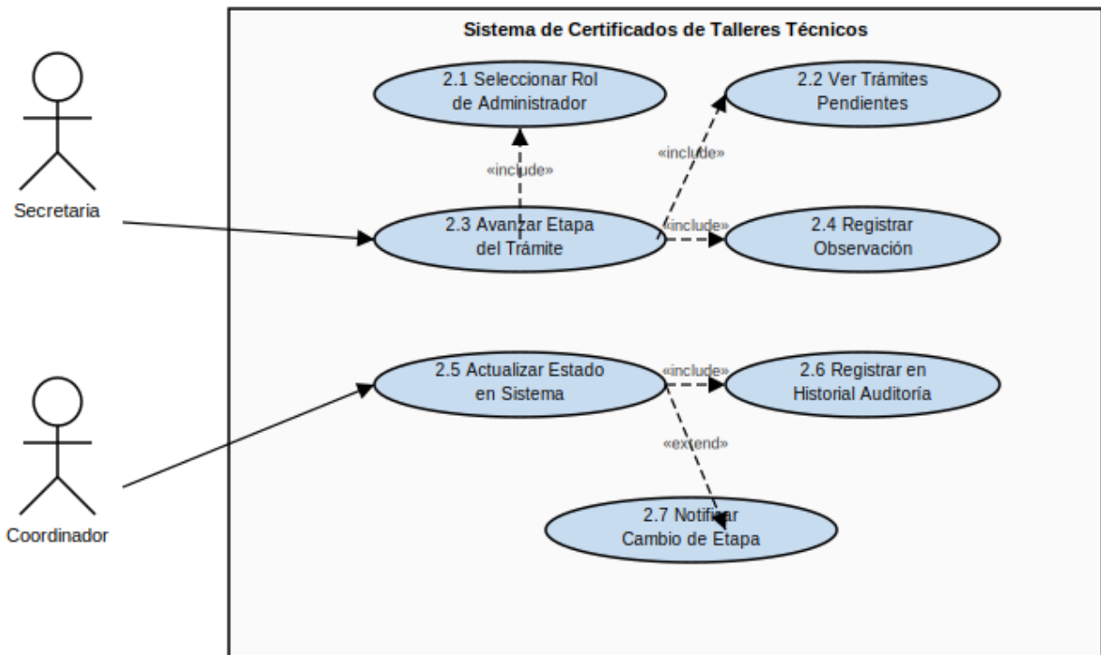
Figura 2.1: Diagrama de caso de uso de la HU 02
