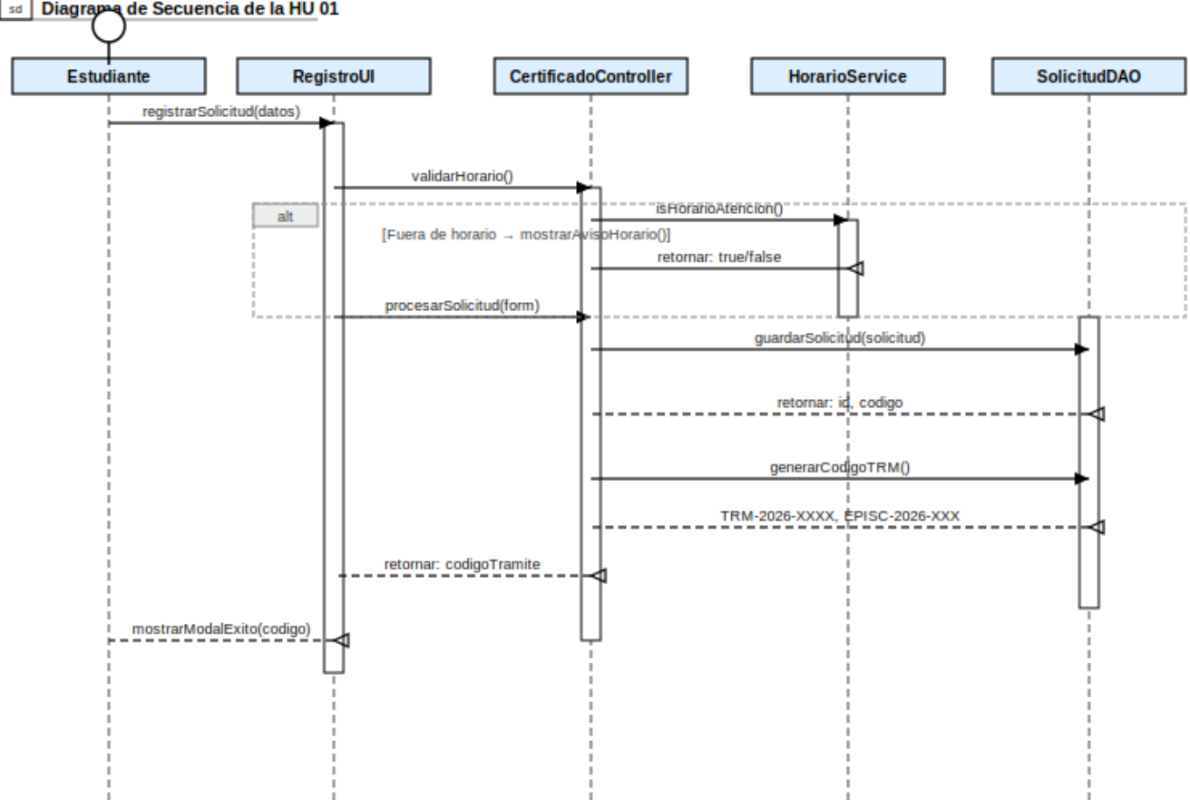
Figura 1.2: Diagrama de secuencia de la HU 01
