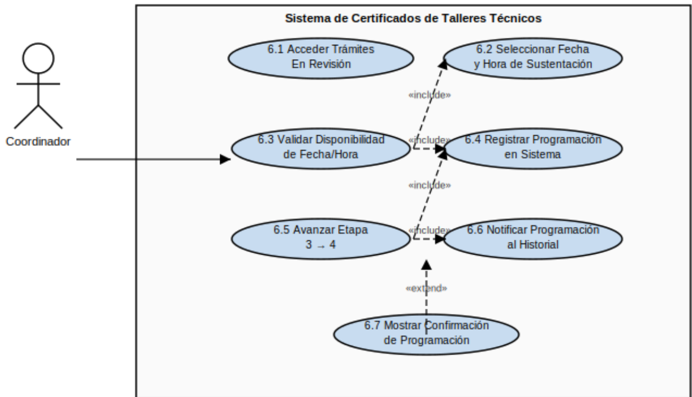
Figura 3.1: Diagrama de caso de uso de la HU 06
