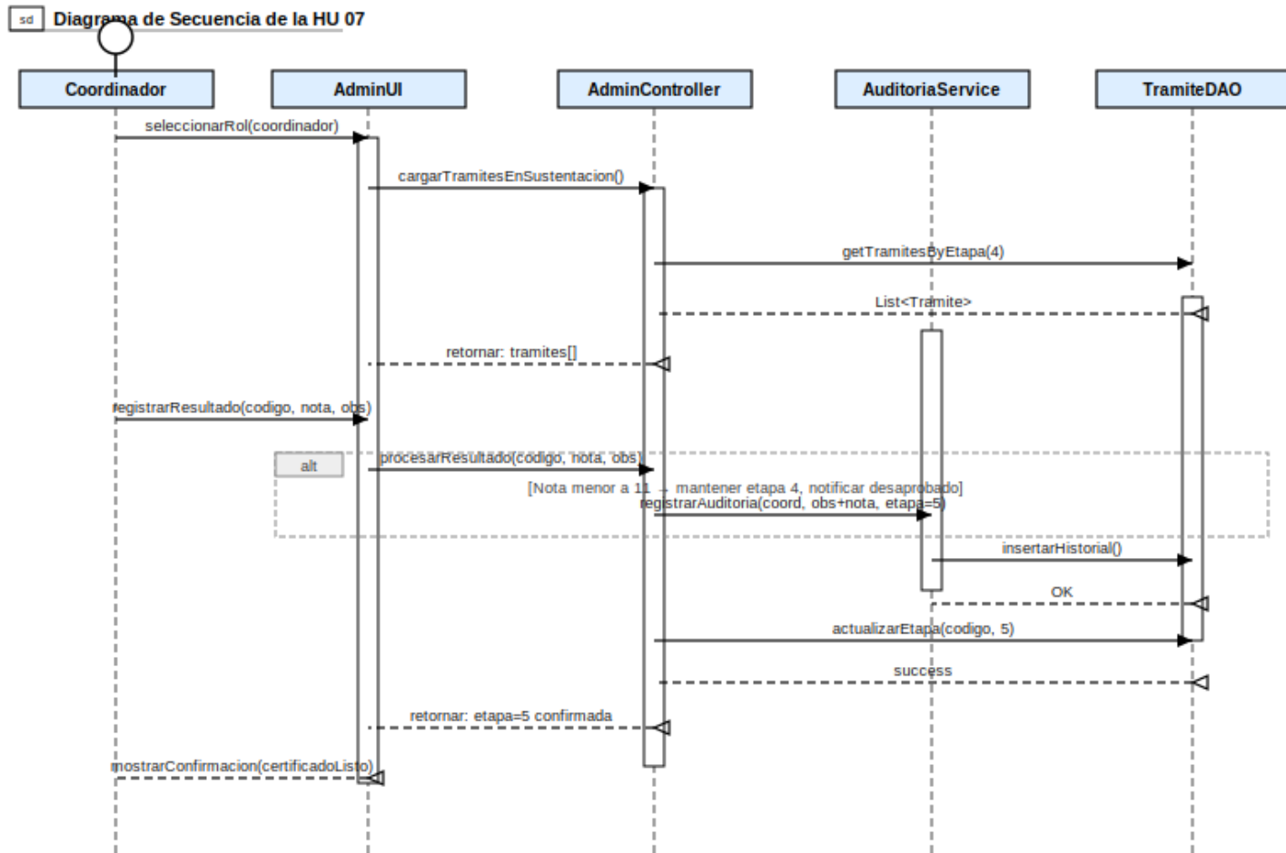
Figura 4.2: Diagrama de secuencia de la HU 07
