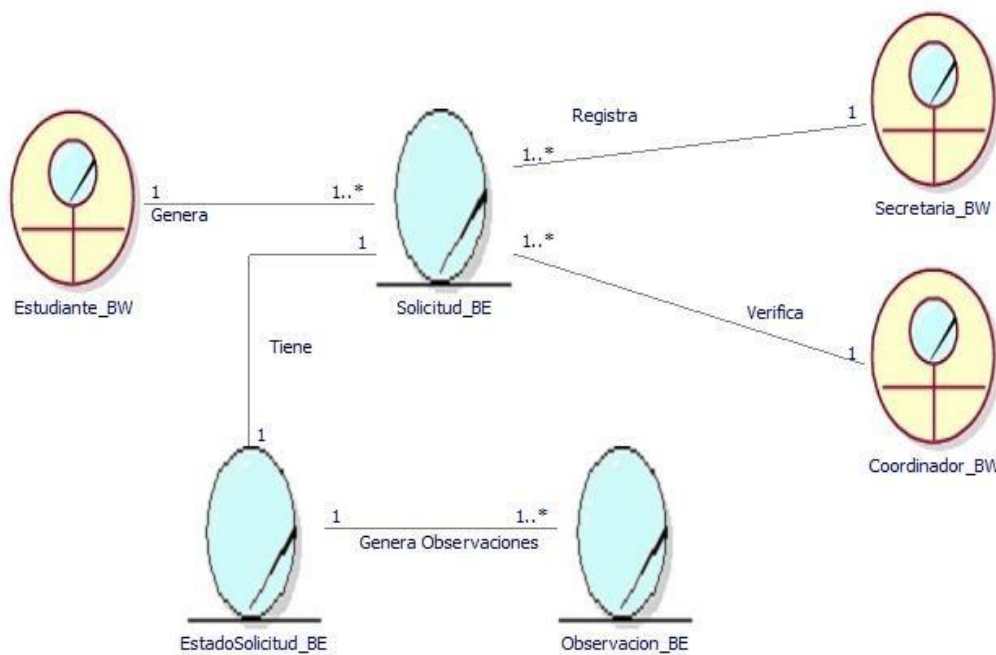
Figura 3. Diagrama de Clases de CUN Gestión de Certificados
