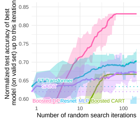
FIGURE 1 – Précisions normalisées de différents classifieurs sur des données tests nouvelles. Les performances sont agrégées pour 16 tâches de classification difficiles. On observe en rose que les performances de notre classifieurs Boosted DPDT sont supérieures à celles des autres modèles apres quelques itérations de recherche d’hyperparamètres.
