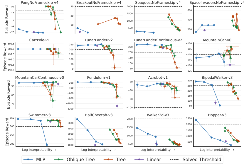
FIGURE 2 – Compromis performances-interprétabilité de différentes classes de politiques de décision pour différents PDMs standards. On peut voir qu’il n’existe aucune classe de politique qui domine les autres sur tous les PDMs testés. Par exemple, sur Swimmer, ce sont les arbres de décision qui ont le meilleur compromis performances-interprétabilité, tandis que sur la version continue du MountainCar, ce sont les politiques linéaires.
