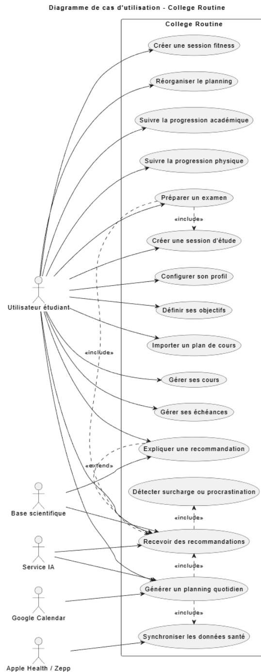
FIGURE 2 – Diagramme de cas d'utilisation - College Routine
