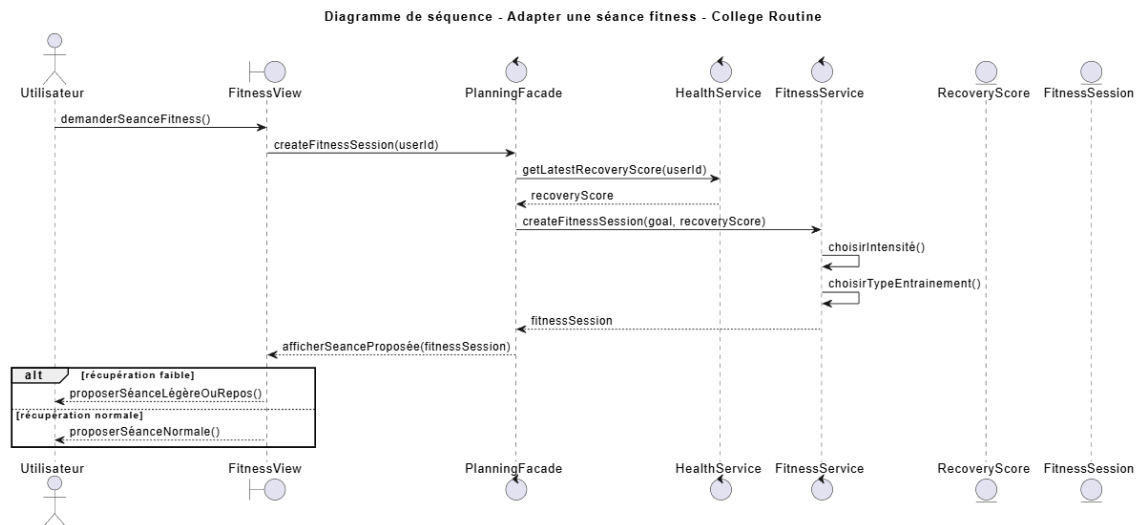
FIGURE 6 – Diagramme de séquence - Adapter une séance fitness - College Routine
