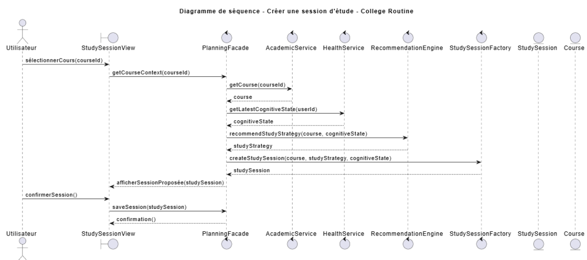
FIGURE 5 – Diagramme de séquence - Créer une session d'étude - College Routine
