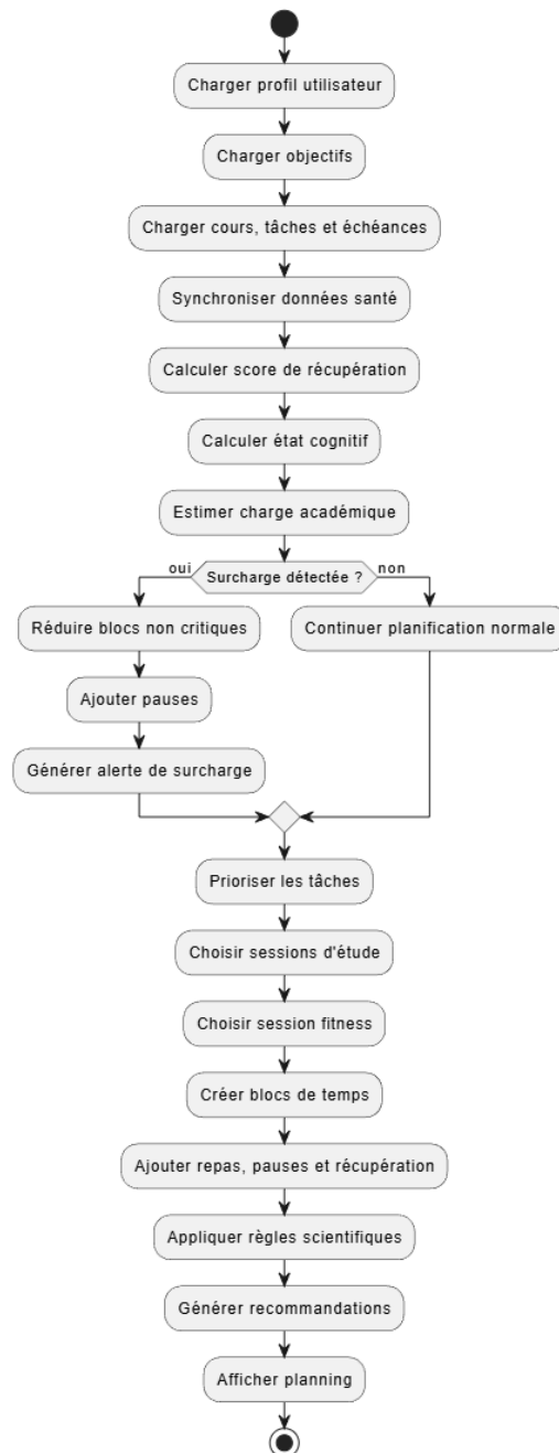
Diagramme d'activité - Génération du planning quotidien - College Routine
