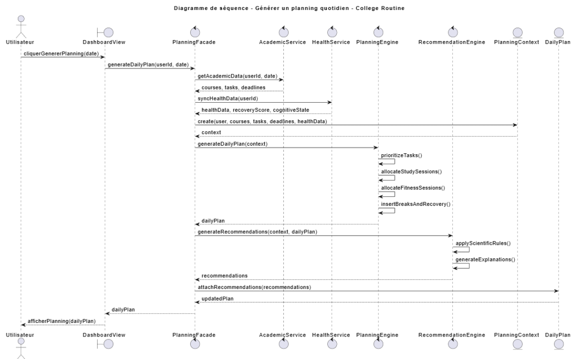
FIGURE 4 – Diagramme de séquence - Générer un planning quotidien - College Routine
