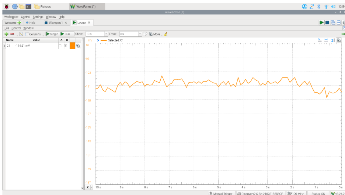
図 9 埋没条件（深さ 64 mm）におけるセンサ応答波形
