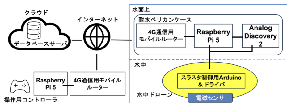
図 2 システム構成図
