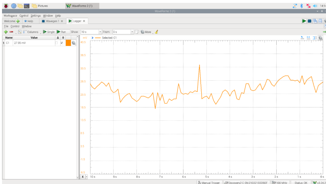
図 10 埋没条件（深さ 30 mm）におけるセンサ応答波形
