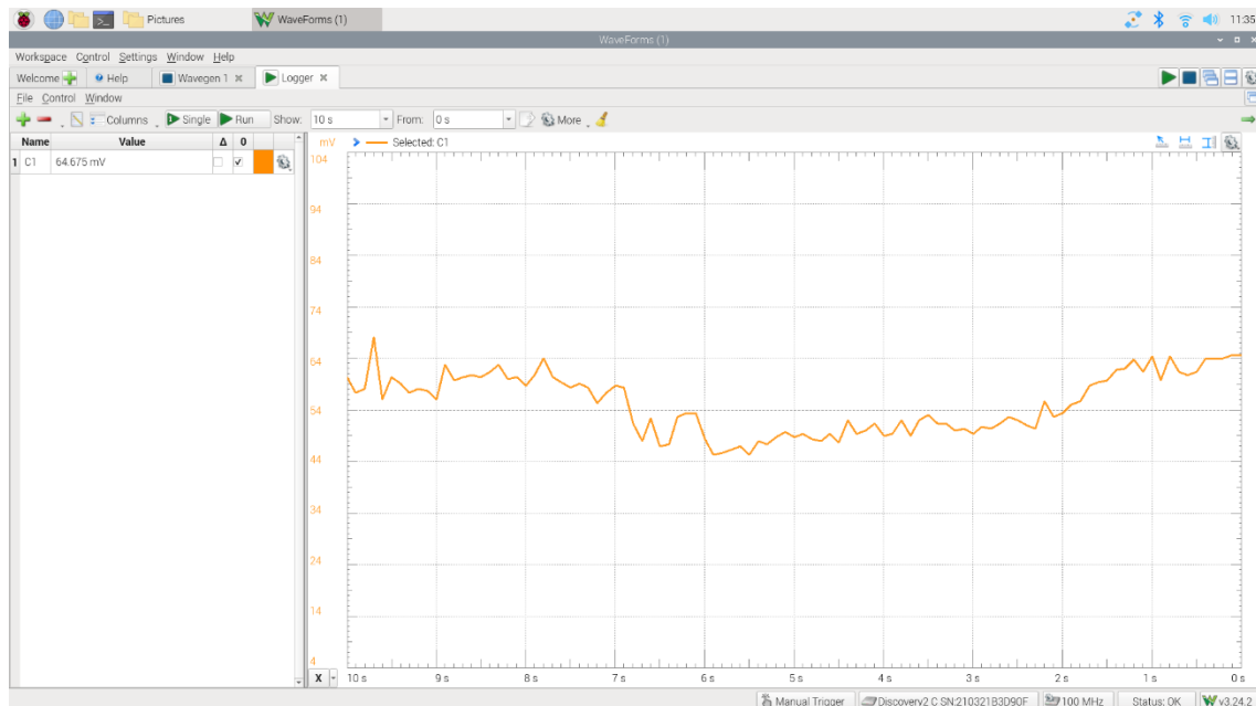
図 15 人工海水環境（基本条件）におけるセンサ応答波形
