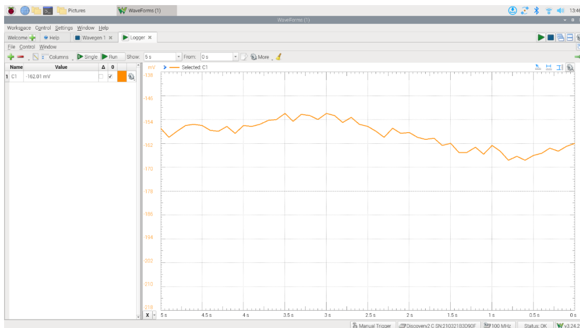
図 13 対照実験（アクリル板）におけるセンサ応答波形
