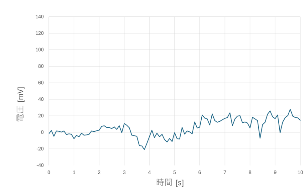
図 18 プール実験におけるセンサ応答波形
