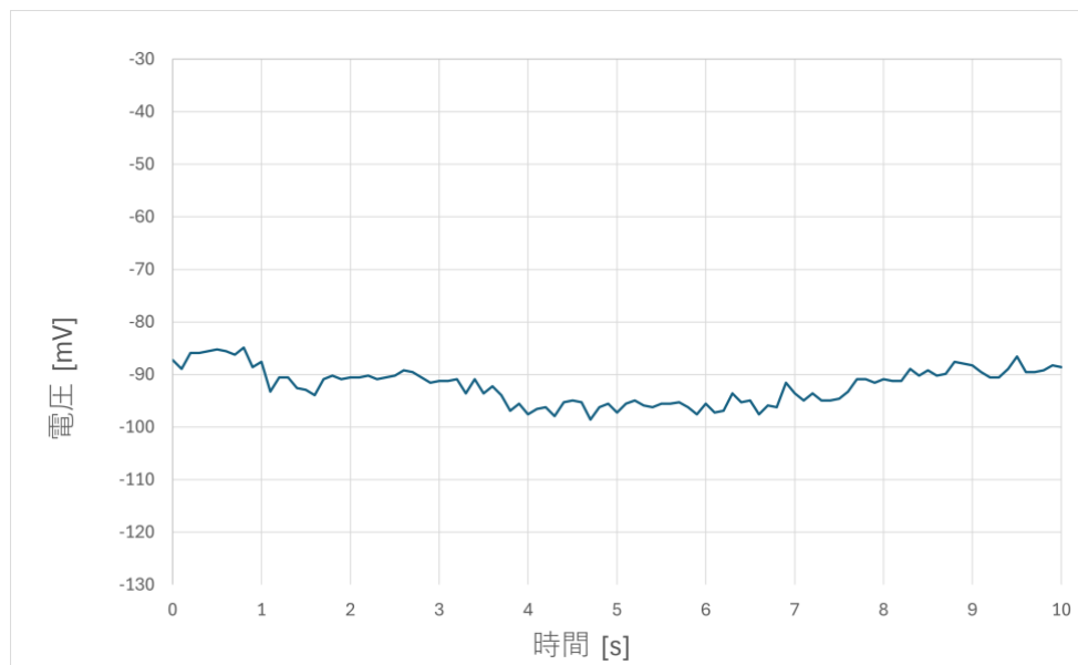
図 13 オフセット条件 (50 mm) におけるセンサ応答波形
