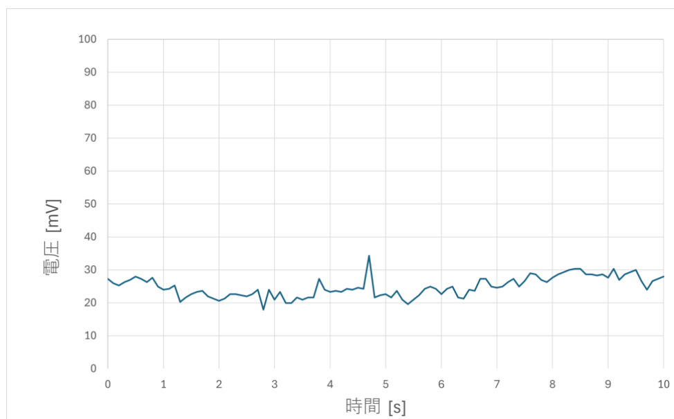
図 11 埋没条件（深さ 30 mm）におけるセンサ応答波形
