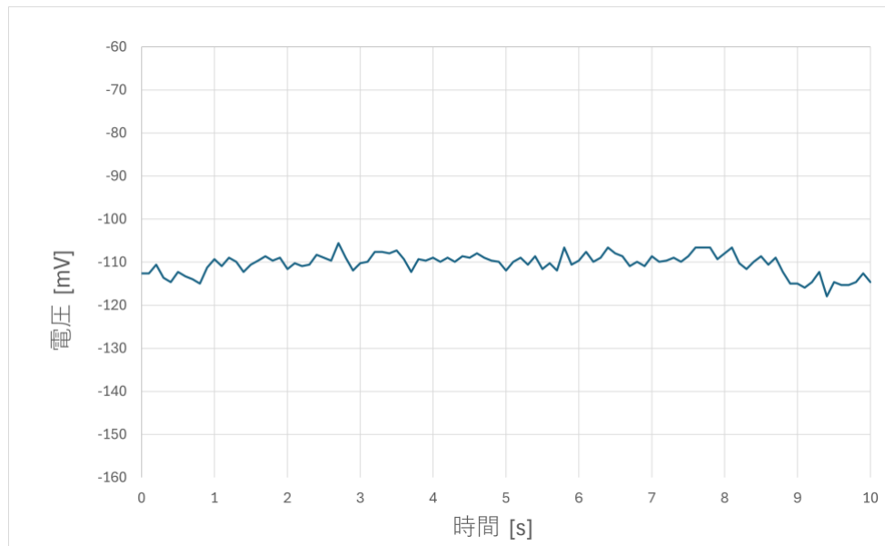
図 10 埋没条件（深さ 64 mm）におけるセンサ応答波形
