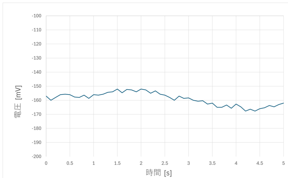
図 14 対照実験（アクリル板）におけるセンサ応答波形
