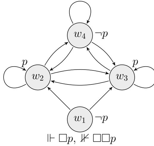
شكل 51.3: نموذج مبرهنة 51.35.
