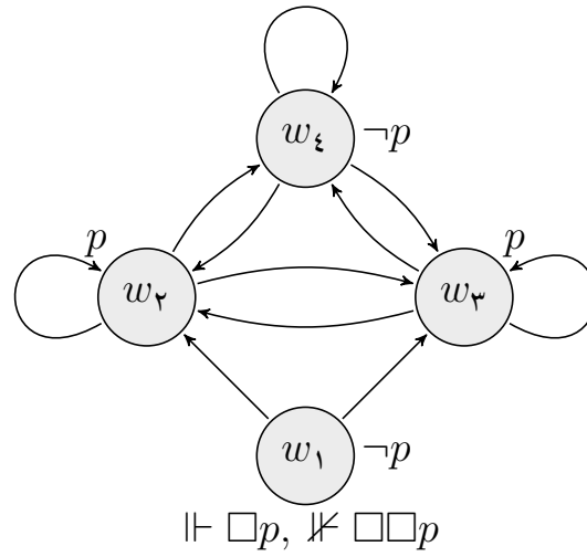
شكل 51.3: نموذج مبرهنة 51.35.
