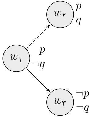
شكل 49.1: نموذج بسيط.
