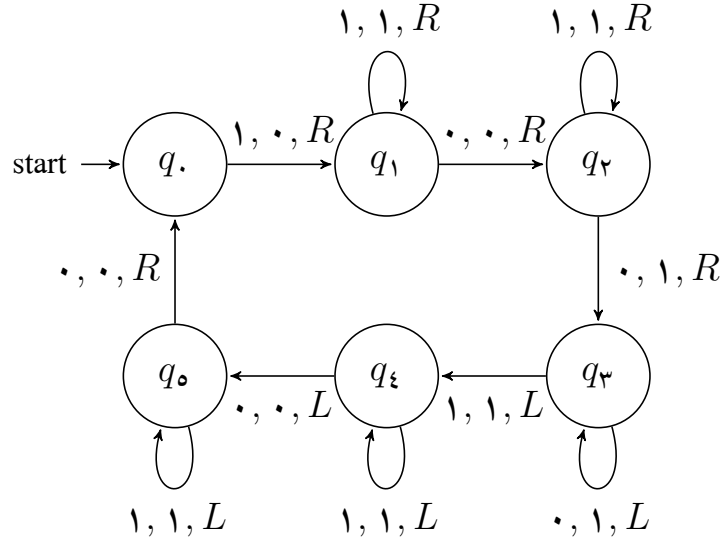
شكل 31.2: آلة مضاعفة
