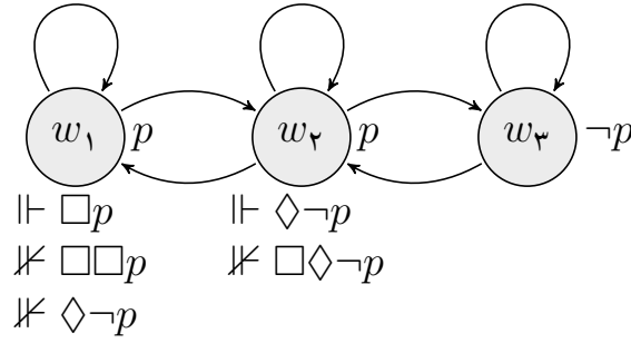
شكل 51.2: نموذج مبرهنة 51.34.
