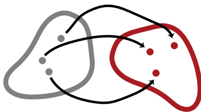
FIGURE 3.4 – Une fonction bijective fait correspondre de manière unique les éléments de l'ensemble d'arrivée à ceux du domaine.
