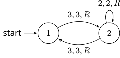
આકૃતિ 29.2: માનક સમ મશીન
