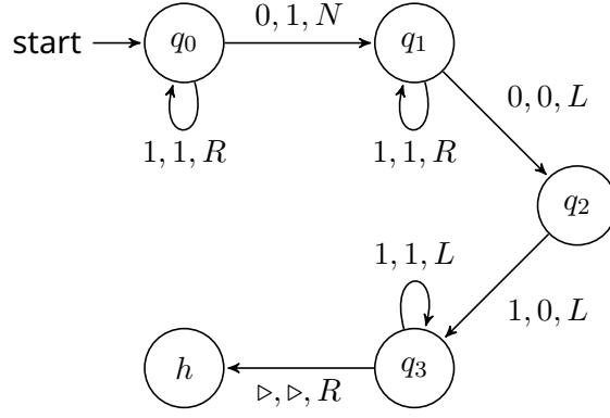
આકૃતિ 28.6: શિસ્તબદ્ધ સરવાળાનું મશીન
