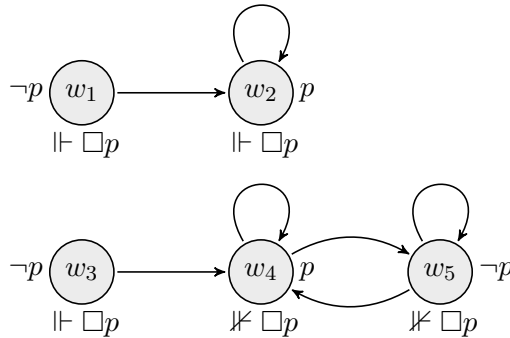
આકૃતિ 56.2: સિરિયલ અને યુક્લિડિયન નિદર્શન.
