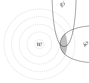
આકૃતિ 66.4: અસત્ય પ્રતિતથ્યાત્મક વિધાન; વિરુદ્ધ પરિણામવાળું પણ અસત્ય
