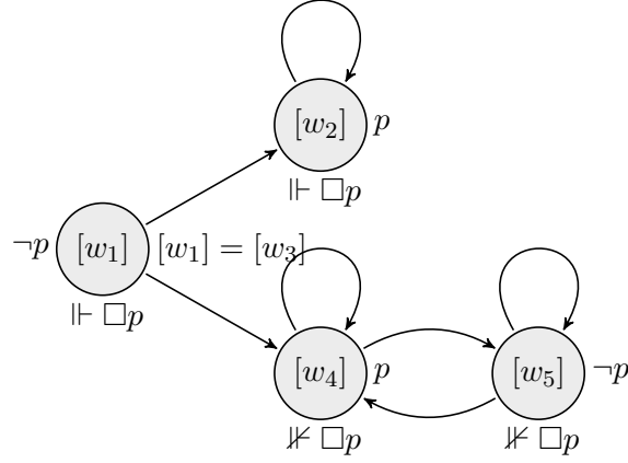
આકૃતિ 56.3: આકૃતિ 56.2ના નિદર્શનનું ફિલ્ટ્રેશન.
