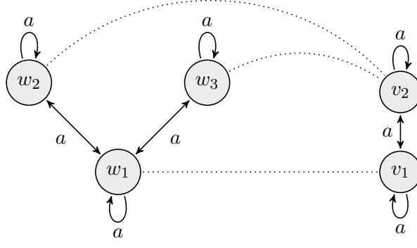
આકૃતિ 60.2: બે દ્વિઅનુકરણ-સમાન નિદર્શો.
