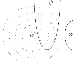
આકૃતિ 66.3: રિક્તતાને કારણે સત્ય પ્રતિતથ્યાત્મક વિધાન
