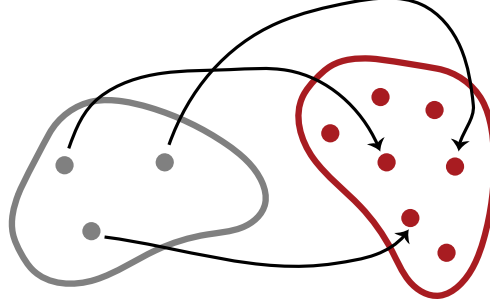
આકૃતિ ૩.૨: વ્યાપ્ત વિધેયના સહપ્રદેશનો દરેક ઘટક તેની કિંમત હોય છે.
