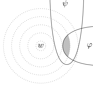
આકૃતિ 66.2: રિક્તતા વગર સત્ય પ્રતિતથ્યાત્મક વિધાન
