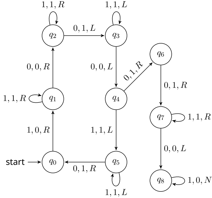
આકૃતિ 28.4: f(x) = 2x ગણતું મશીન
