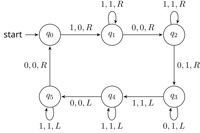
આકૃતિ 28.2: બમણું કરનાર મશીન
