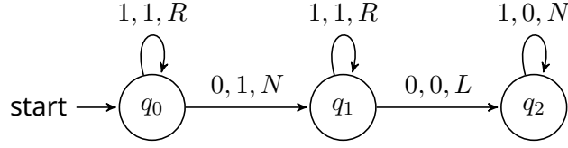
આકૃતિ 28.3: f(x, y) = x + y ગણતું મશીન
