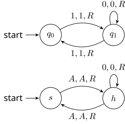
આકૃતિ 29.1: સમ મશીનનાં બે રૂપ
