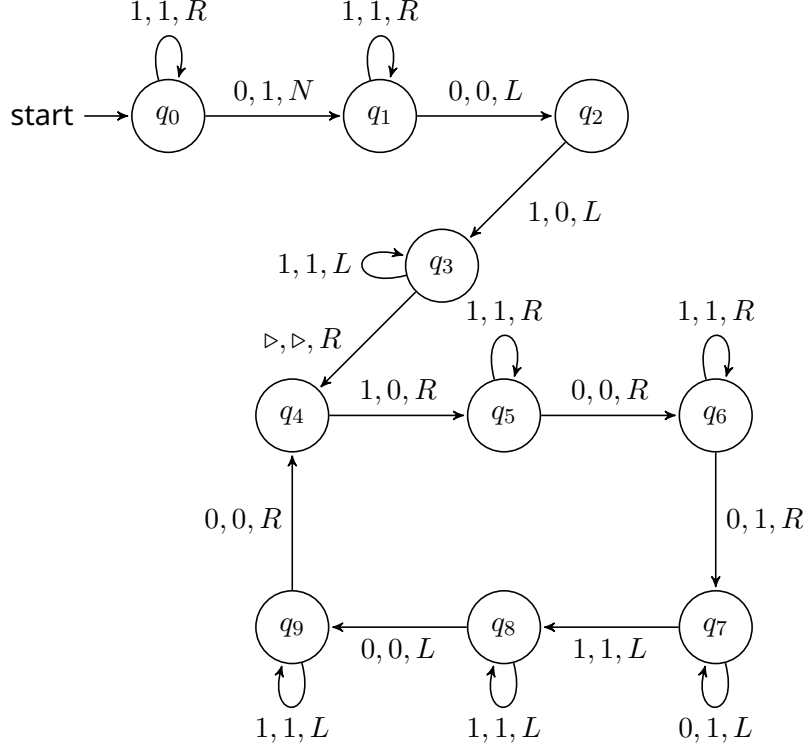
આકૃતિ 28.7: સરવાળાનું અને બમણું કરનાર મશીન જોડવાં
