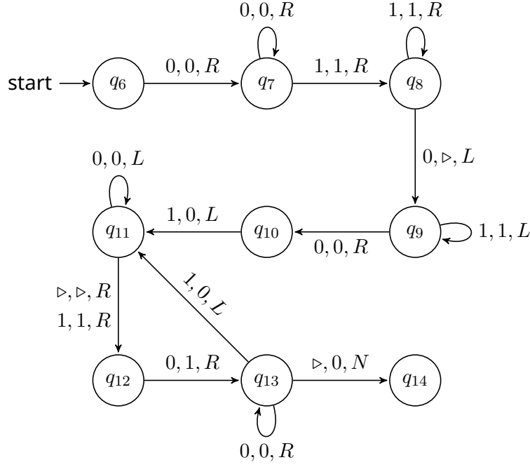
આકૃતિ 28.5: 1ના સમૂહને ડાબે ખસેડવું
