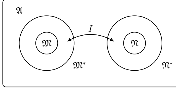
આકૃતિ 25.1: આંતરિક આંશિક એકરૂપતા ધરાવતી સંરચના ધ્ર.
