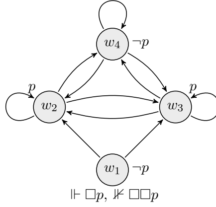
આકૃતિ 54.3: પ્રમેય 54.35 માટેનું નિદર્શન.
