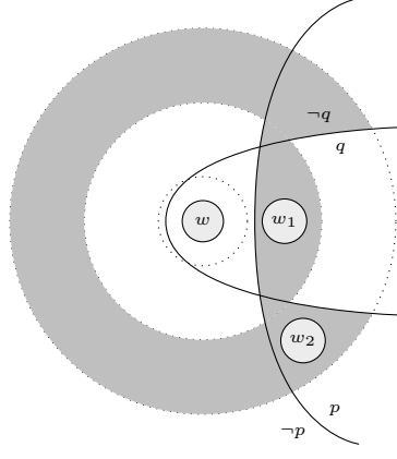
આકૃતિ 66.8: પ્રતિપક્ષી રૂપાંતરનું પ્રત્યુદાહરણ
