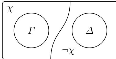
આકૃતિ 24.1: \chi , \Gamma અને \Delta ને પૃથક કરે છે
