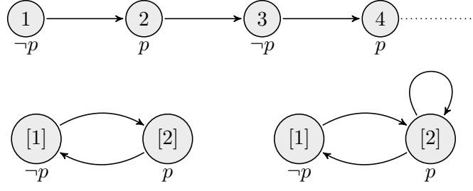
આકૃતિ 56.1: અનંત નિદર્શન અને તેનાં ફિલ્ટ્રેશનો.
