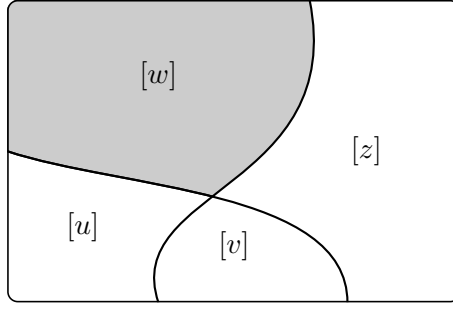
આકૃતિ 53.2: સામ્ય વર્ગોમાં W નું વિભાજન.
