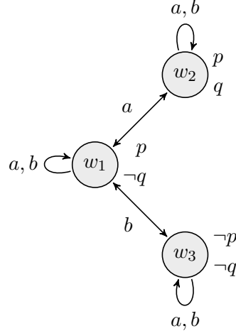
આકૃતિ 60.1: એક સરળ જ્ઞાનસંબંધી નિદર્શ.
