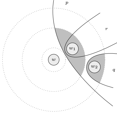
આકૃતિ 66.7: પૂર્વપક્ષને મજબૂત કરવાના નિયમનું પ્રત્યુદાહરણ
