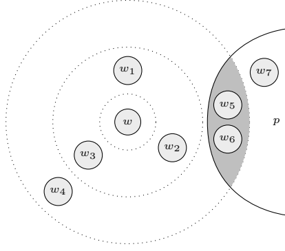
આકૃતિ 66.1: ગોળા-નિદર્શનો આલેખ
