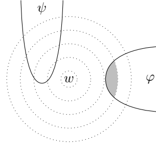
આકૃતિ 66.5: અસત્ય પ્રતિતથ્યાત્મક વિધાન; વિરુદ્ધ પરિણામવાળું સત્ય
