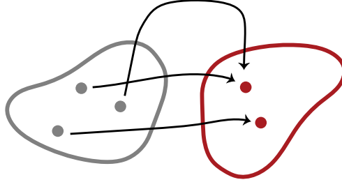
આકૃતિ ૩.૨: વ્યાપ્ત વિધેયના સહપ્રદેશનો દરેક ઘટક તેની કિંમત હોય છે.
