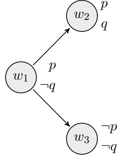
આકૃતિ 52.1: સરળ નિદર્શન.
