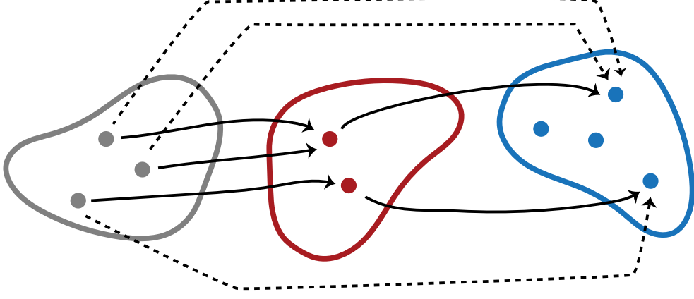
આકૃતિ ૩.૫: બે વિધેયો f અને g નું સંયોજન g \circ f .
