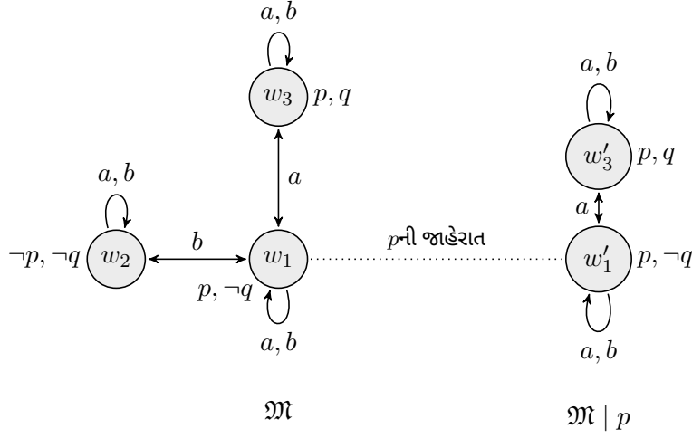
આકૃતિ 60.3: p ની જાહેર જાહેરાત પહેલાં અને પછી.
