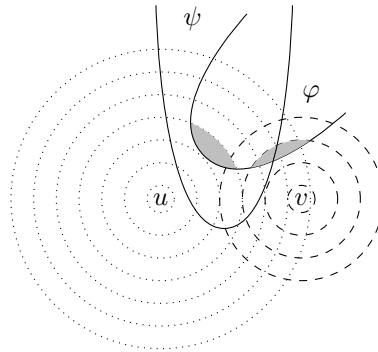
આકૃતિ 66.6: સંજોગાધીન પ્રતિતથ્યાત્મક વિધાન
