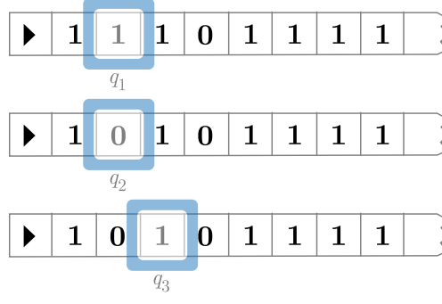
આકૃતિ 28.1: પોતાનો પ્રોગ્રામ ચલાવતું ટ્યુરિંગ મશીન.
