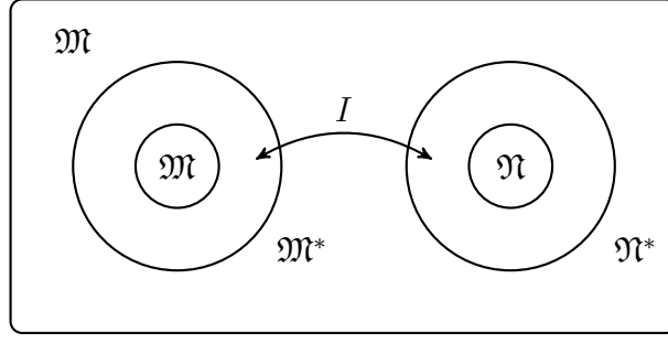
படம் 22.1: உள்ளார்ந்த பகுதி ஓரினச்சார்புடன் கூடிய கட்டமைப்பு \mathcal{M} .
