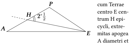
extremitas perigea P. Inclinatio 2° 1/2 diametri subtendit oculo observatoris terrestris angulum HEA 1° 2' in extremitate apogea, HEP 6° 22' in perigea. (5) Respectu centri Terrae 1° 46' in extremitate apogea, 4° 5' in perigea.
