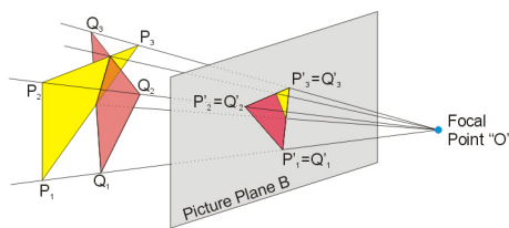
Gambar 93: Diagram perspektif dengan sinar-sinar proyeksi yang menghubungkan objek, pusat proyeksi, dan bidang gambar
