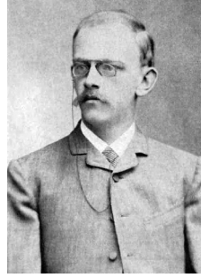
Gambar 60: David Hilbert (1862–1943)
