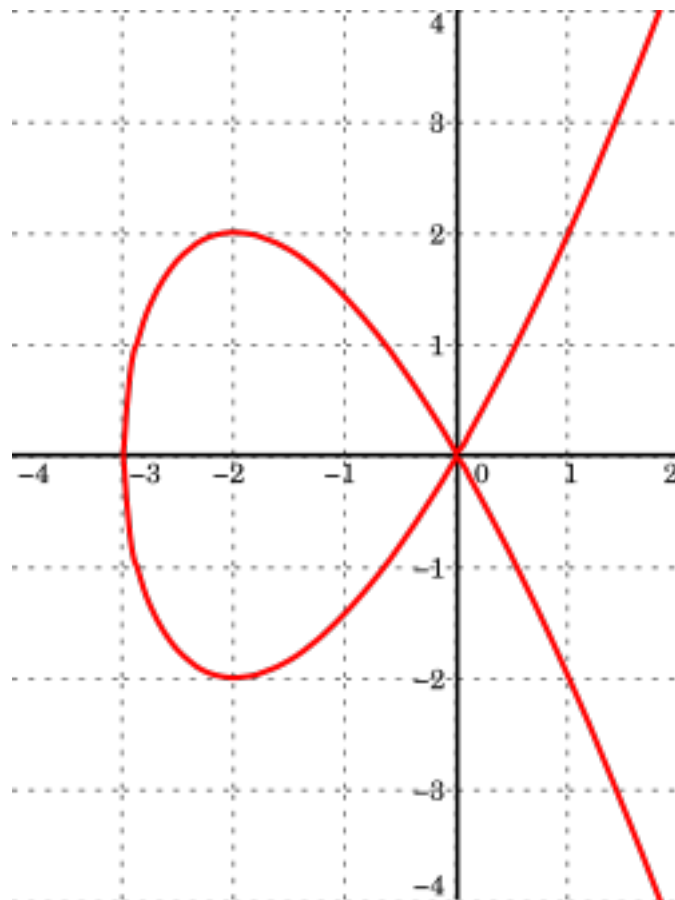
Gambar 8: Kubik Tschirnhausen
