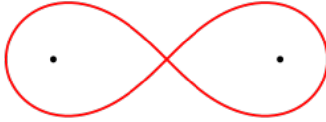
Gambar 99: Lemniskat Bernoulli. Karya Zorgit, domain publik.
