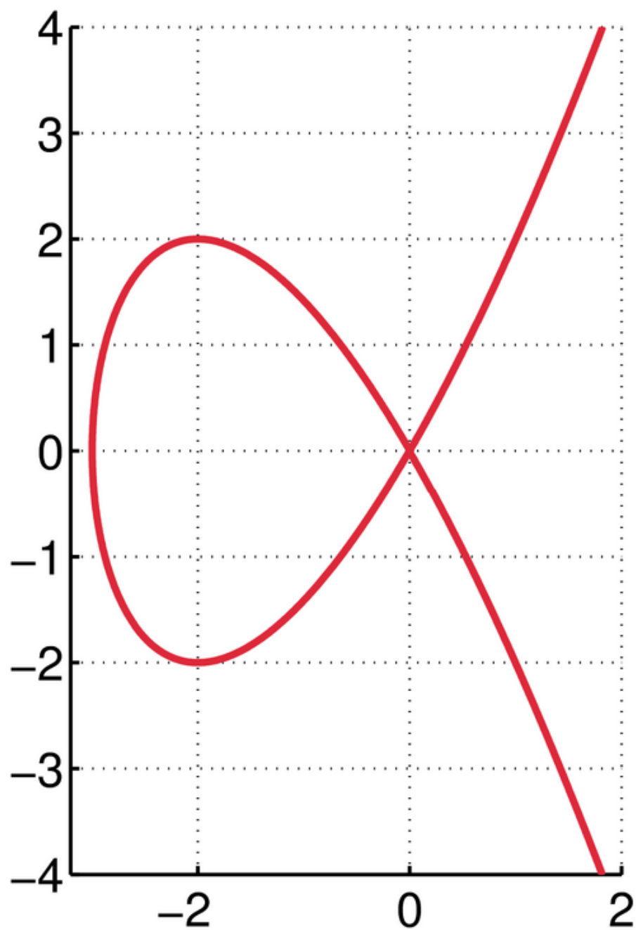
Gambar 100: “Kubik Tschirnhausen” menurut keterangan sebaris kursus. Karya Oleg Alexandrov, domain publik.
