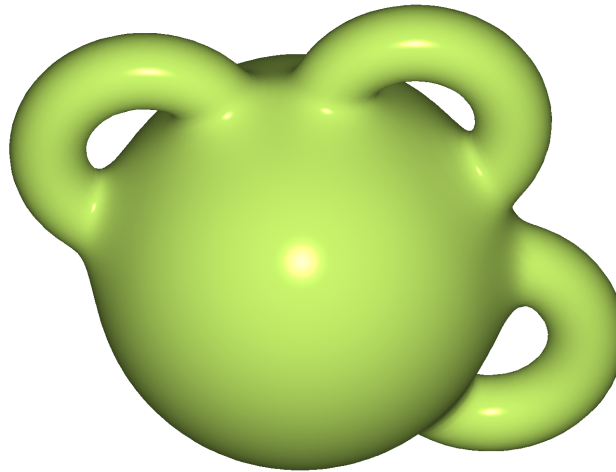
Gambar 98: Ilustrasi sfera dengan tiga gagang
