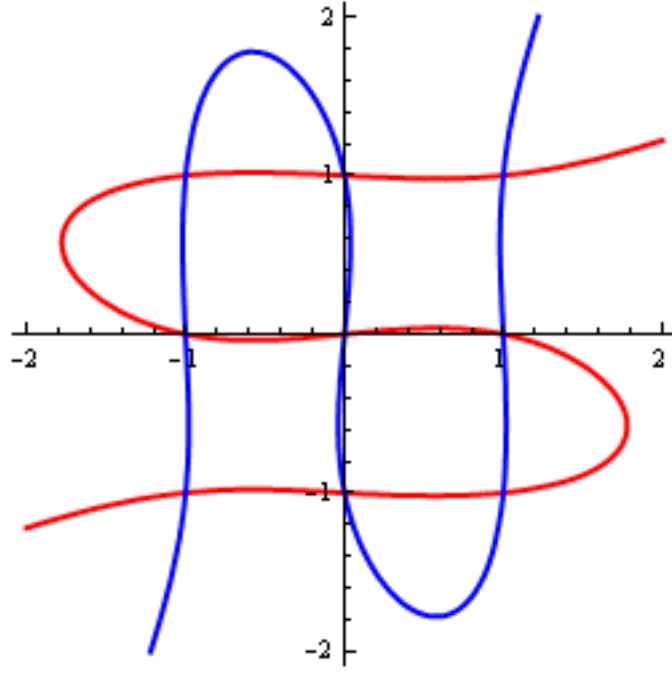
Gambar 101: Dua kurva kubik. Karya Hack, dibuat dengan Mathematica 6, domain publik.
