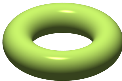
Gambar 96: Ilustrasi torus sebagai permukaan dengan satu gagang
