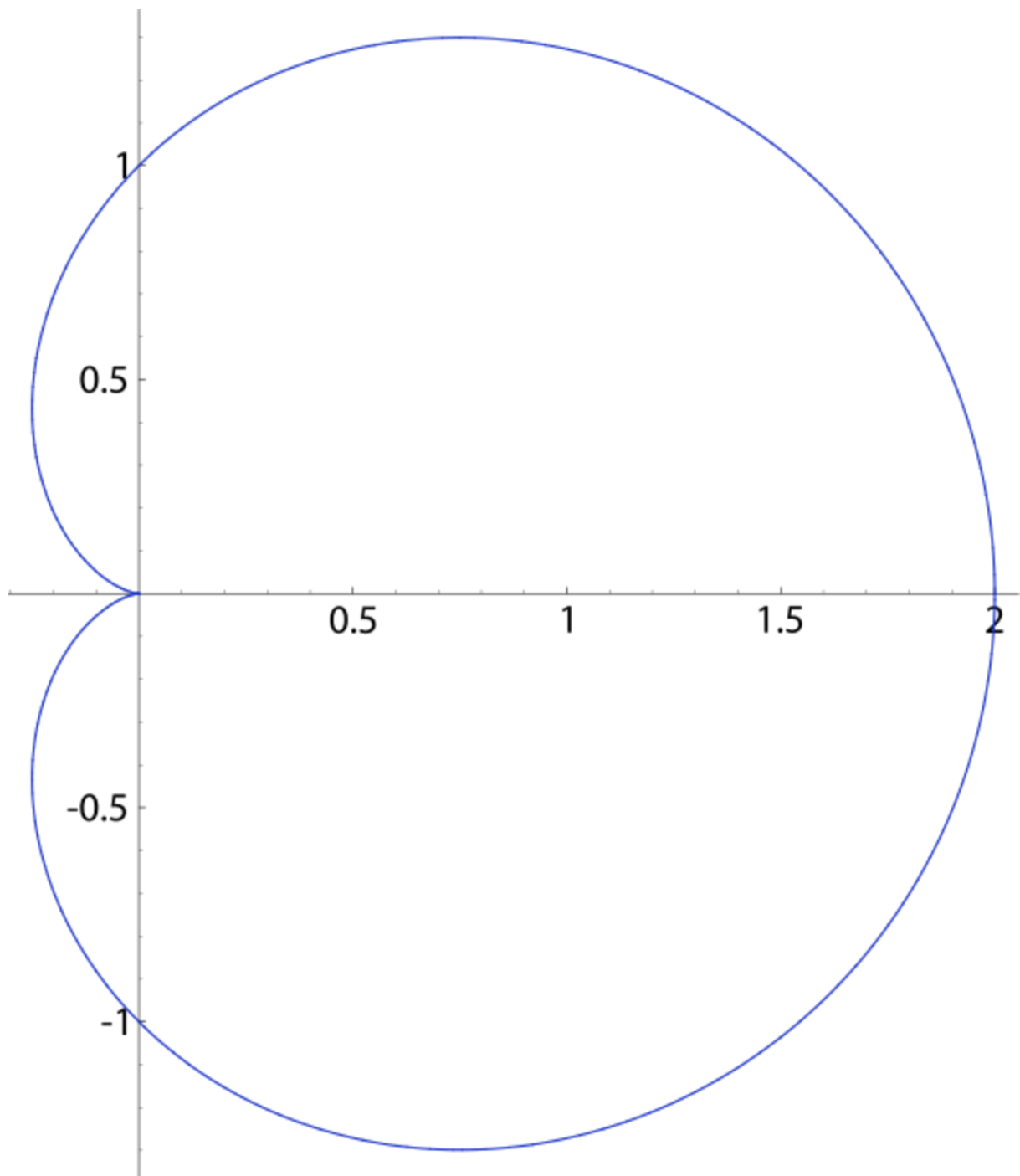
Gambar 83: Grafik kardioid simetris dengan titik runcing di sisi kiri dan lengkungan membulat di sisi kanan
